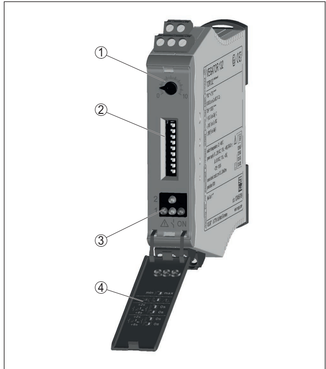
Fig. 3: Elementos de indicación y ajuste
