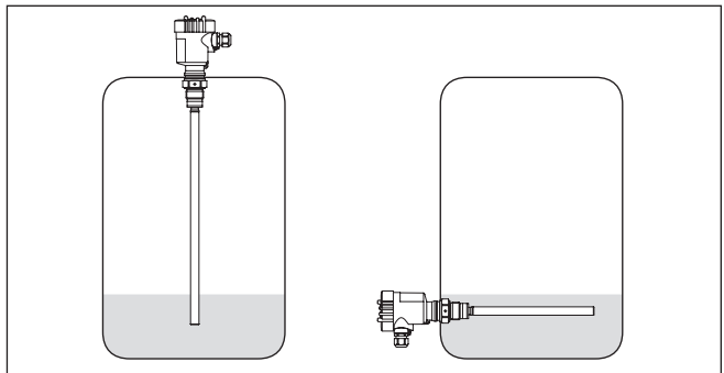
Fig. 7: Ejemplos de aplicación protección contra marcha en seco con interruptor de nivel conductivo
