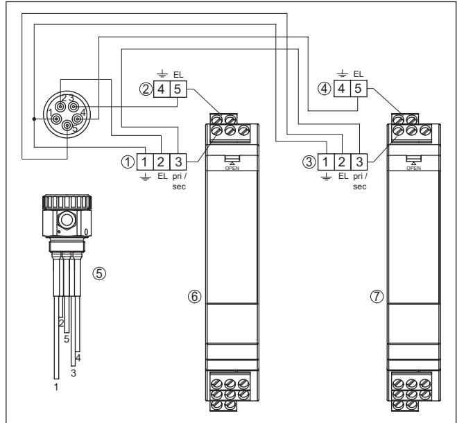
Fig. 2: Esquema de conexión VEGATOR 132
