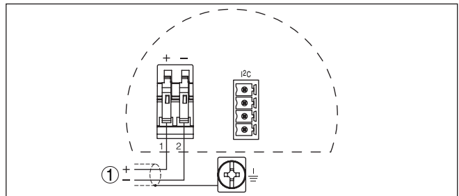
Abb. 3: Anschlussplan - Zweikammergehäuse
