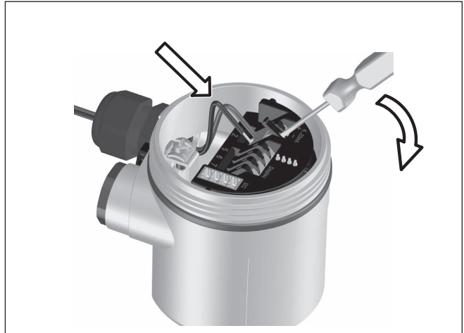
Abb. 1: Anschlusschritte 6 und 7
