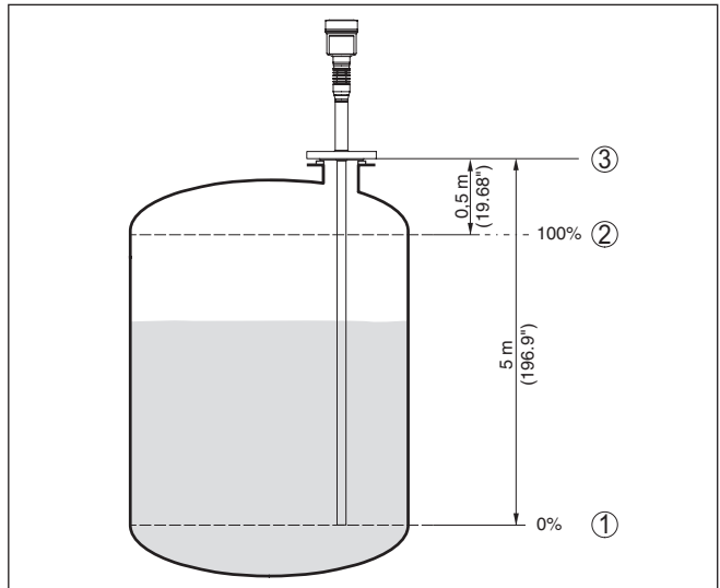
Abb. 5: Parametrierbeispiel Min.-/Max.-Abgleich
