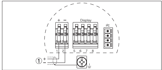
Abb. 2: Anschlussplan - Einkammergehäuse
