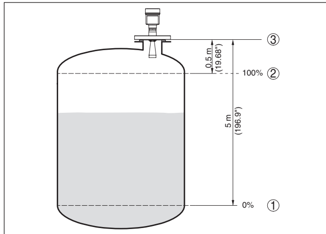
Abb. 5: Parametrierbeispiel Min.-/Max.-Abgleich
