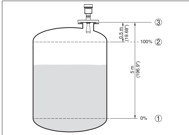
Abb. 6: Parametrierbeispiel Min.-/Max.-Abgleich
