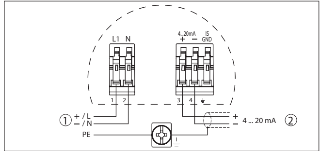
Abb. 3: Anschlussplan - Zweikammergehäuse
