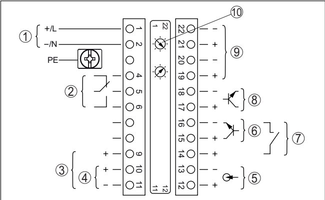
插图. 9: 非防爆仪表和带有非自安全电流输出出口的仪表上的电子部件和接线腔
