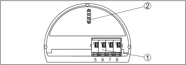
插图. 14: 非防爆仪表和带有非自安全电流输出出口的仪表上的操作和接线腔
