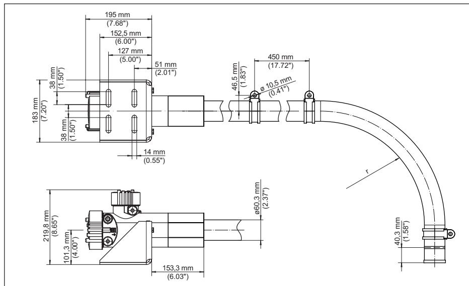
插图. 30: FIBERTRAC 32 带随附的安装配件
