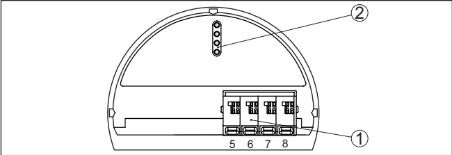
插图. 10: 非防爆仪表和带有非自安全电流输出出口的仪表上的操作和接线腔
