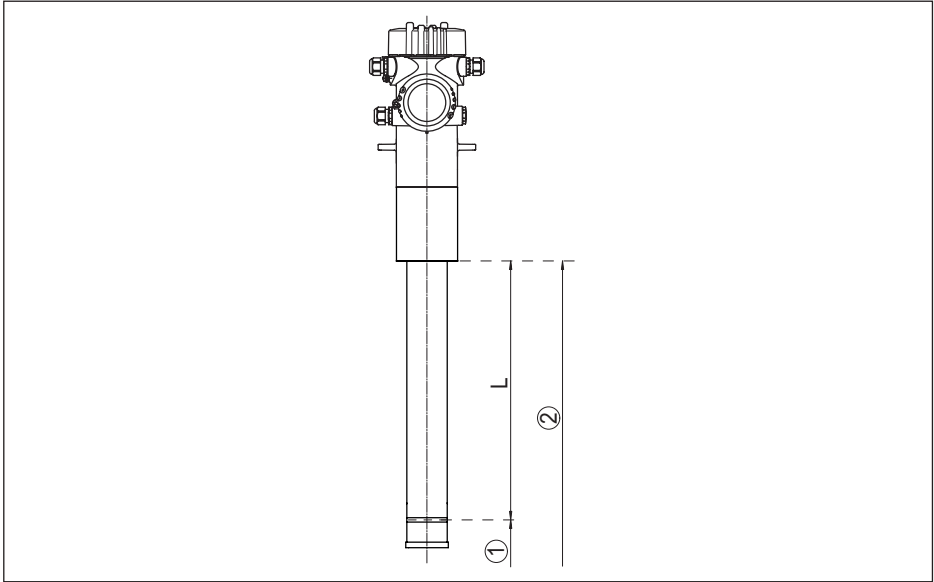
插图. 27: 有关输入值的信息 1 最小物位 (红色的标记线) 2 最大物位 L 测量范围 (仪表的订购长度)
