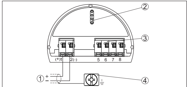
插图. 16: 在带有自安全电流输出出口的仪表上的操作和接线腔 (防爆 (ia))
