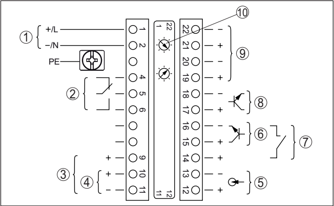
插图. 13: 非防爆仪表和带有非自安全电流输出出口的仪表上的电子部件和接线腔
