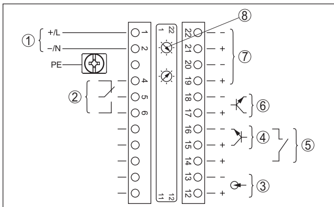
插图. 11: 在带有自安全电流输出出口的仪表上的电子部件和接线腔 (防爆 (d))
