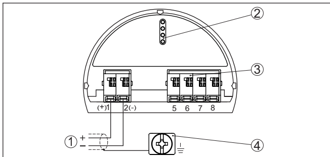
插图. 12: 在带有自安全电流输出出口的仪表上的操作和接线腔 (防爆 (ia))
