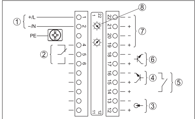
插图. 15: 在带有自安全电流输出出口的仪表上的电子部件和接线腔 (防爆 (d))
