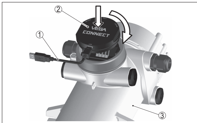
Figura 22: Allacciamento del PC direttamente al sensore tramite adattatore d'interfaccia
