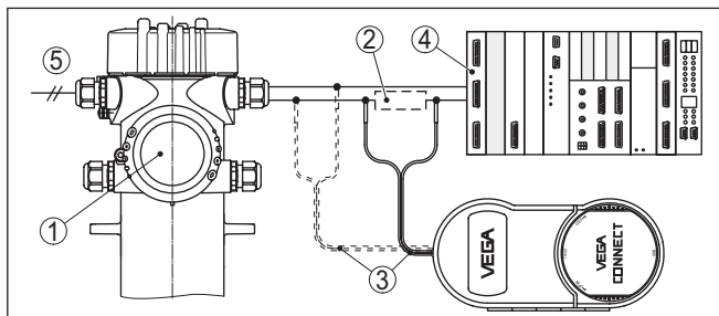
Figura 23: Collegamento del PC via HART alla linea del segnale
