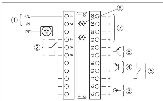
Figura 15: Vano dell'elettronica e di connessione (Ex-d) per apparecchi con uscita in corrente a sicurezza intrinseca
