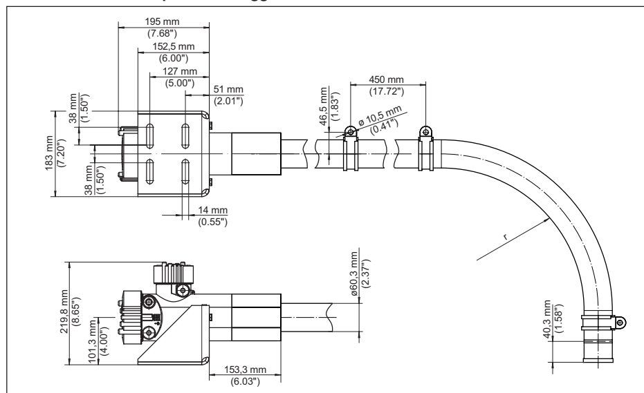
Figura 30: FIBERTRAC 32 con accessori di montaggio in dotazione
