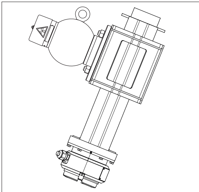
Figura 2: Modulatore gamma (opzionale) per una misura senza interruzioni anche in presenza di radiazioni estranee.
