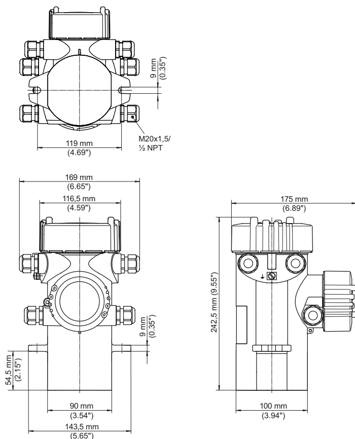
Figura 28: Custodia di alluminio o di acciaio speciale (microfuso)
