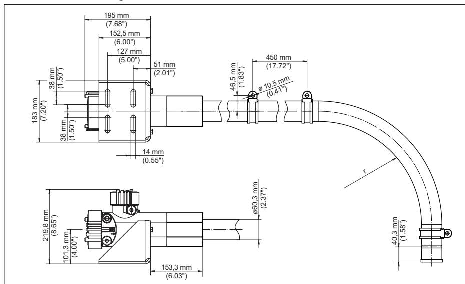
Fig. 29: FIBERTRAC 32 met meegeleverde montage toebehoren
