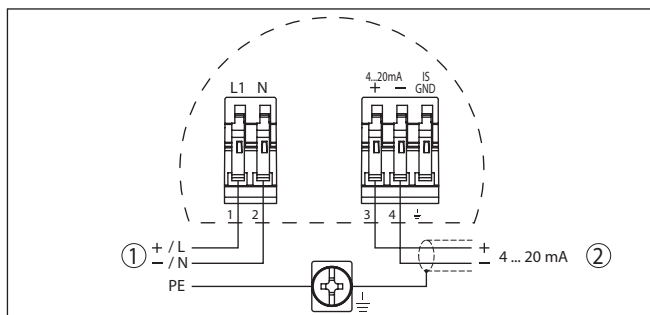
Fig. 4: Aansluitschema - tweekamerbehuizing
