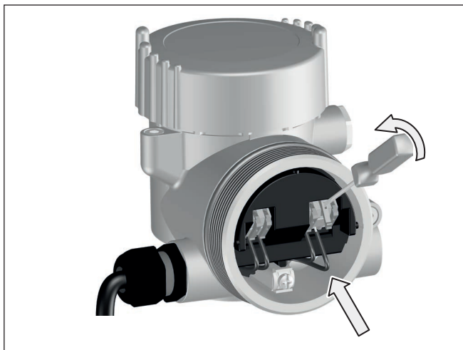
Fig. 3: Aansluitstappen 5 en 6
