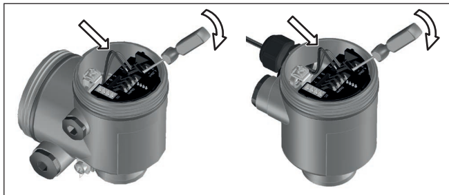
Abb. 3: Anschlussschritte 6 und 7
