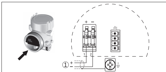
Abb. 5: Anschlussplan - Zweikammergehäuse
