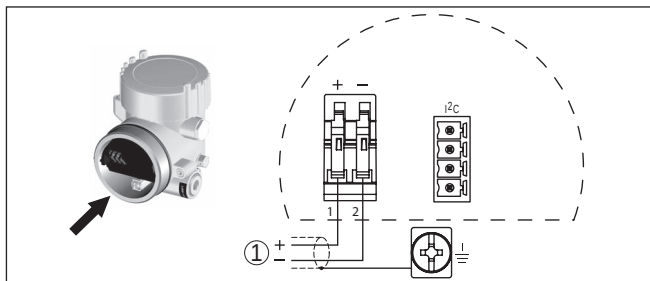
Fig. 5: Aansluitschema - tweekamerbehuizing
