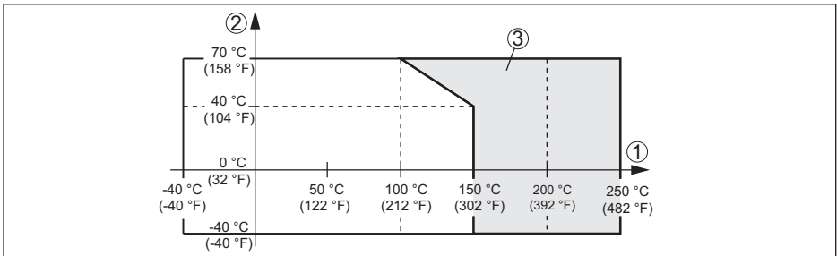
Abb. 1: Umgebungstemperatur - Prozesstemperatur
