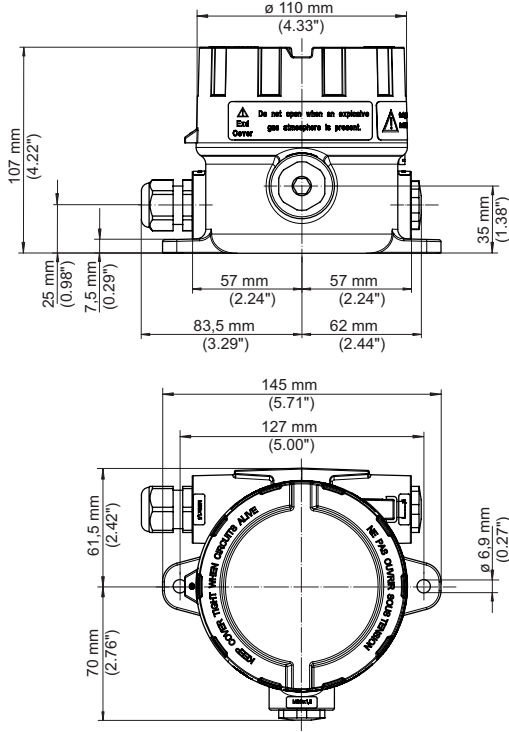
Res. 21: Alüminyum gövdeli PLICSMOBILE B81 ebatları
