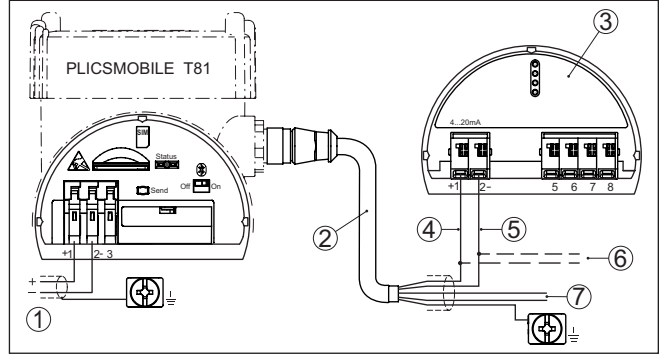
Res. 6: Bağlantı, güç kaynağı ve plics® sensörü
