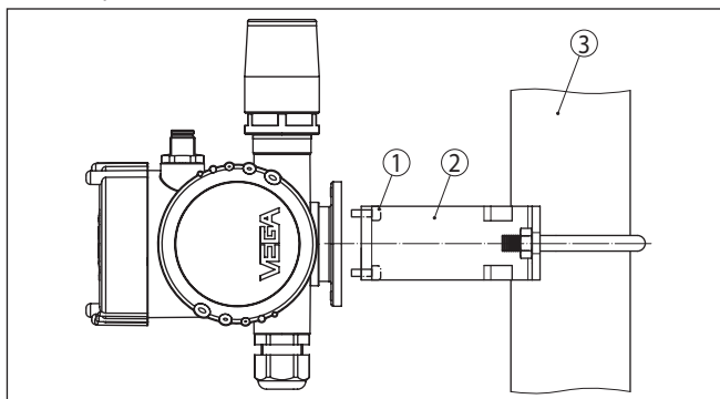
Fig. 4: PLICSMOBILE T81 pour montage sur tuyauterie
