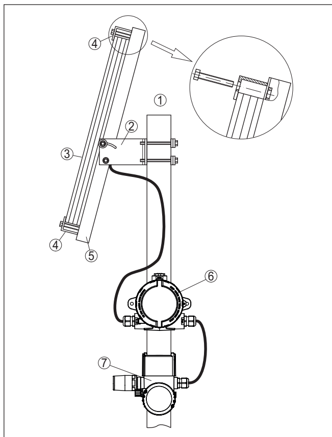
Fig. 13: Montage sur tuyauterie PLICSMOBILE avec module solaire
