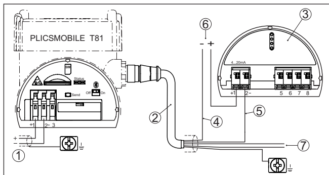
Fig. 10: Raccordement de l'alimentation tension
