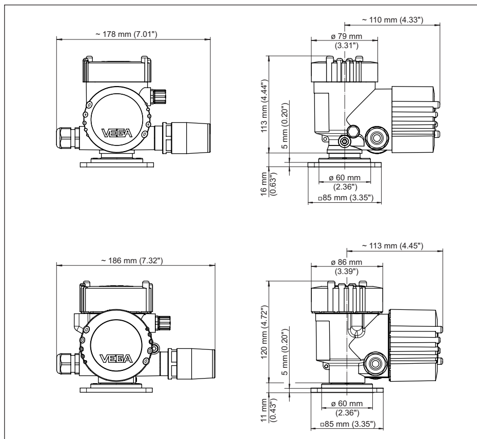
Fig. 20: Dimensions PLICSMOBILE T81 avec boîtier en plastique et boîtier aluminium/acier inoxydable
