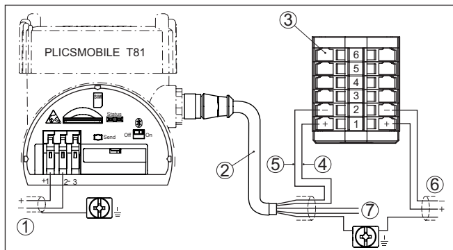
Fig. 7: Raccordement de l'alimentation tension et de la VEGABOX 03
