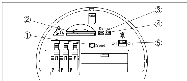
Fig. 14: Éléments de réglage et d'affichage
