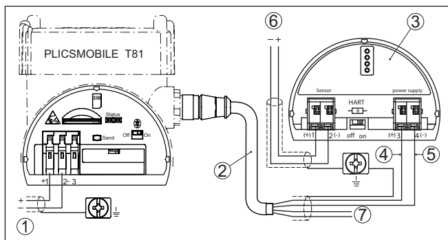
Fig. 8: Raccordement de l'alimentation tension et du VEGADIS 82 HART
