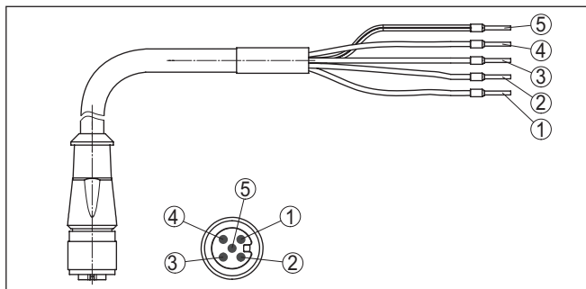
Fig. 9: Affectation des broches du câble de connexion de capteur
