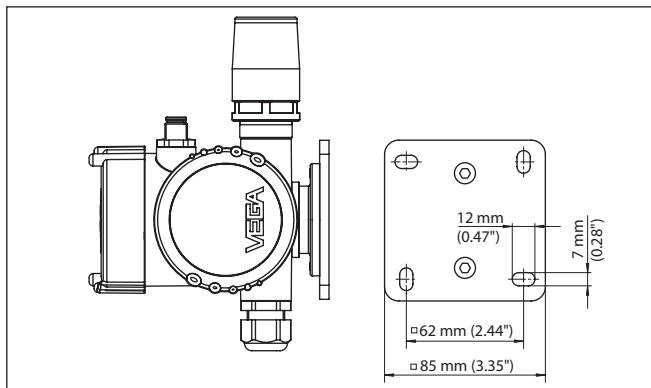
Fig. 2: PLICSMOBILE T81 pour montage mural. Plaque de montage vue de dessous.
