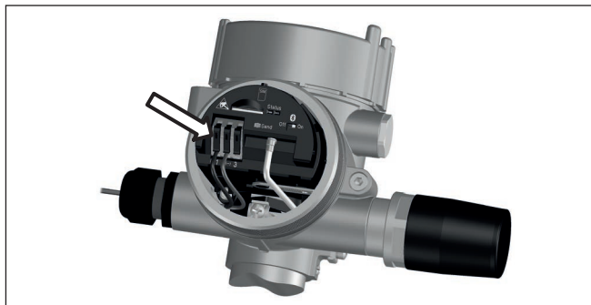
Fig. 5: Étapes de raccordement 4 et 5
