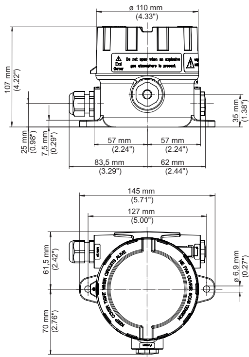
Fig. 21: Dimensions PLICSMOBILE B81 avec boîtier aluminium
