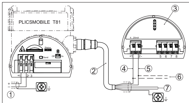
Fig. 6: Raccordement alimentation tension et capteur plics®
