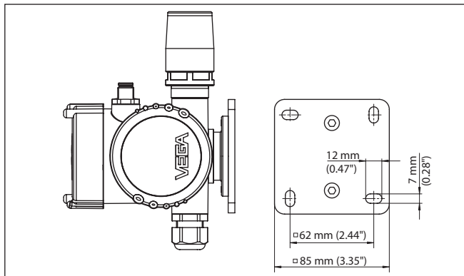
Fig. 2: PLICSMOBILE T81 voor wandmontage. Montageplaat van onderen gezien.
