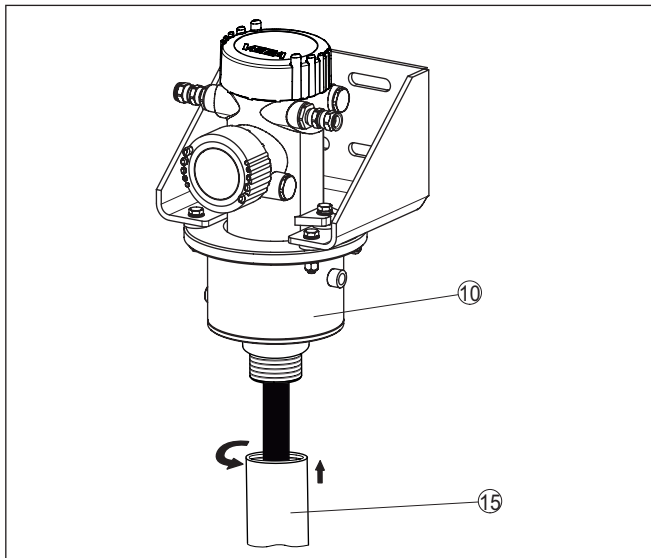
插图. 5: 闪烁体冷却装置的安装
