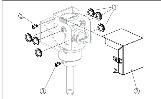
插图. 13: 备件 - 带压缩空气接口 (车间) 的空气冷却装置 - 闪烁体冷却管，带 Conduit 接口
