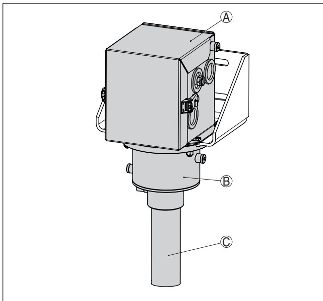
插图 1: 带有固定角的有源气冷系统
