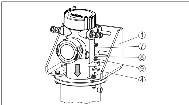
插图. 4: 传感器的安装
