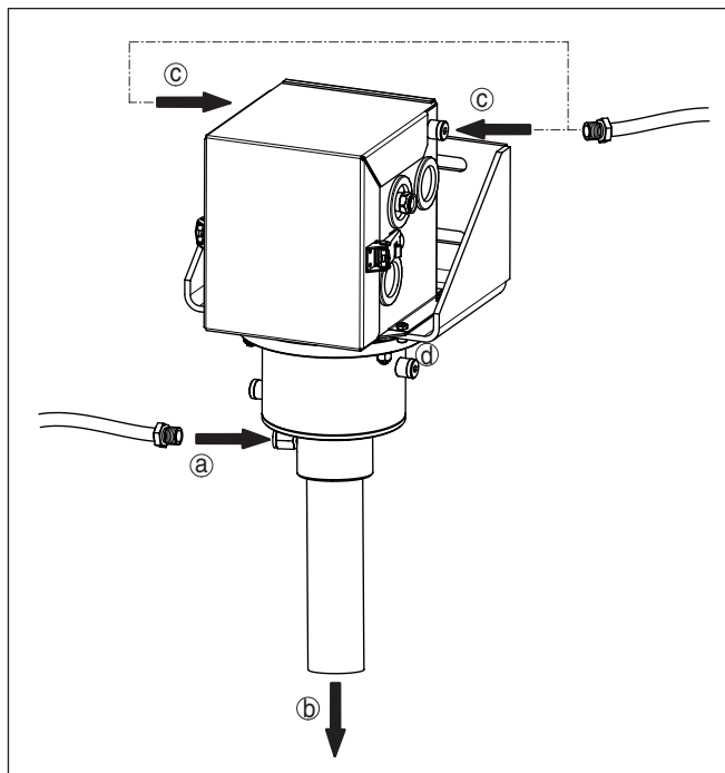
插图. 11: 连接冷却空气管道
