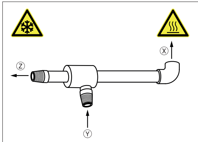
插图. 9: 漩流散热器 (漩涡散热器)
