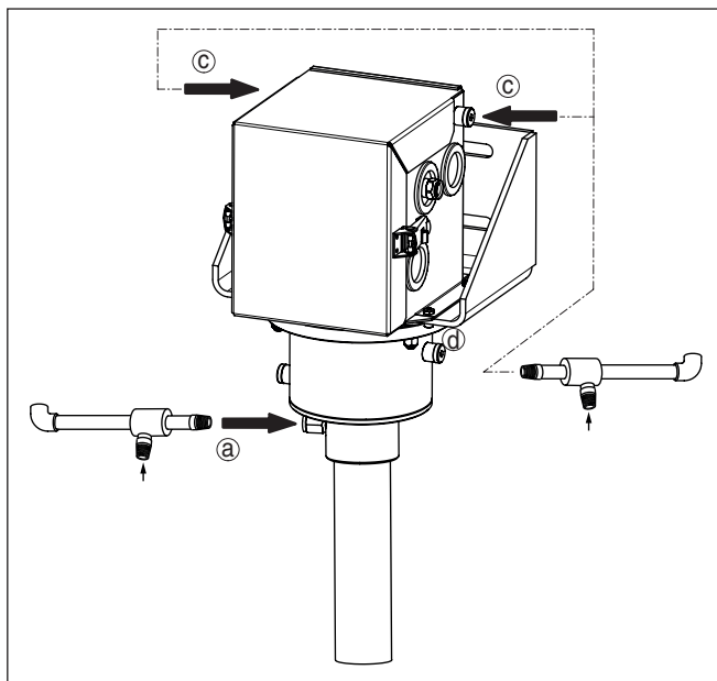
插图. 10: 连接冷气系统 (旋流散热器)
