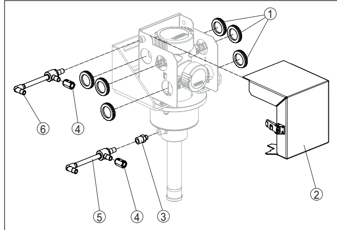
插图. 12: 备件 - 带有旋流散热器的气冷装置 - 闪烁体冷却管，带 Conduit 接口
