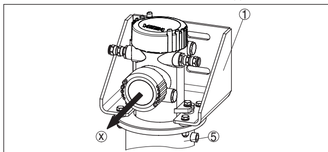
插图. 3: 传感器在固定角上的安装方向
