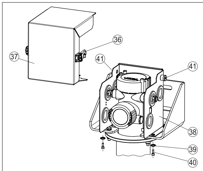
插图. 7: 壳体冷却盒的安装
