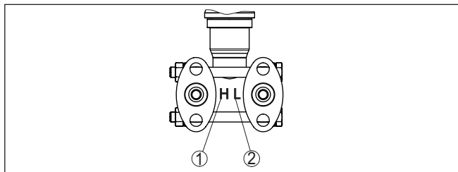
Figura 9: Contrassegno per il lato di alta/bassa pressione sull'unità di processo
