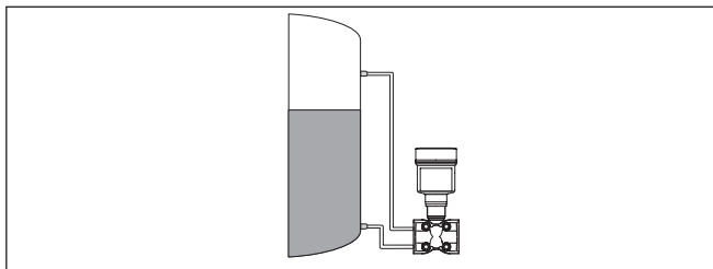
Figura 2: Misura di livello con VEGADIF 85 in un serbatoio in pressione
