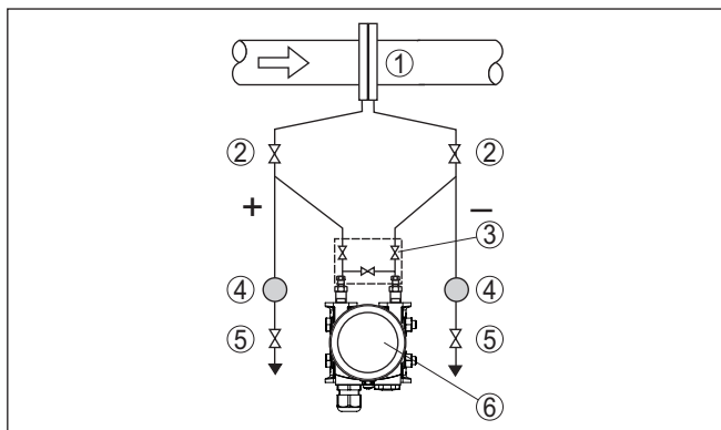
Fig. 18: Meelopstelling bij doorstroommeting in vloeistoffen
