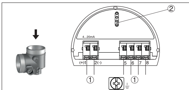
Fig. 31: Elektronicaruimte - Ex-d-tweekamerbehuizing
