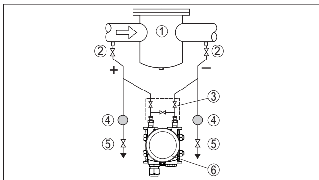
Fig. 21: Meetopstelling bij verschilddrukmeting in vloeistoffen
