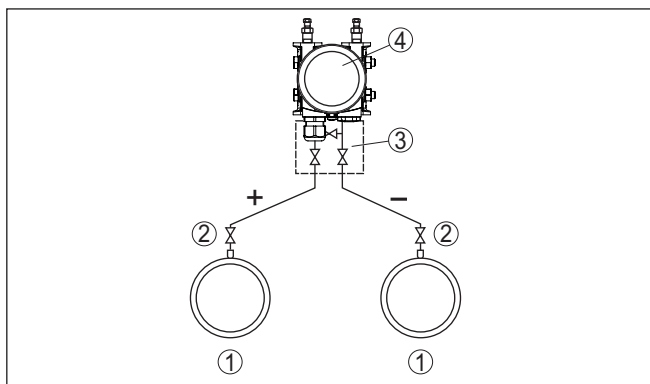
Fig. 19: Meelopstelling bij verschilddrukmeting tussen twee leidingen in gasen en dampen
