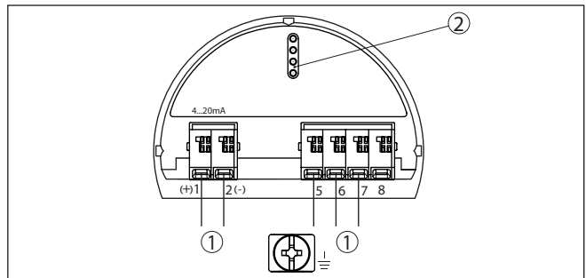
Fig. 3: Compartiment électronique - boîtier à deux chambres
