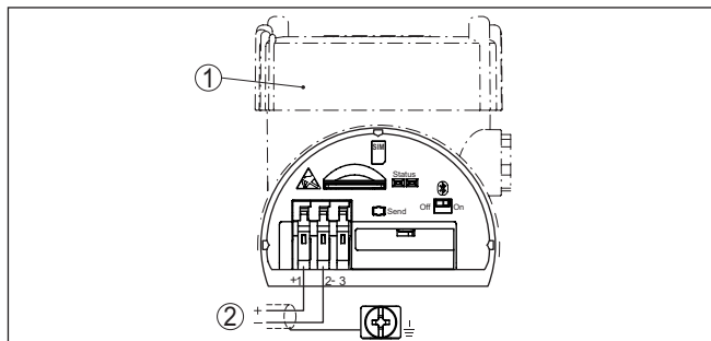
Abb. 3: Anschluss der PLICSMOBILE 81-Spannungsversorgung
