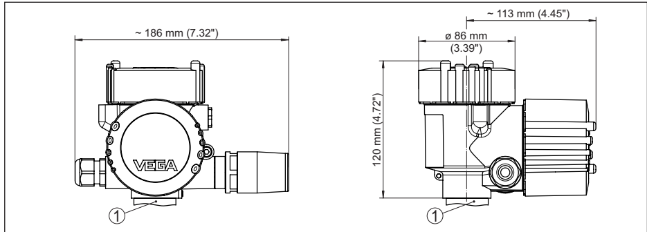
Abb. 12: Maße PLICSMOBILE 81 mit VA-/Aluminiumgehäuse
