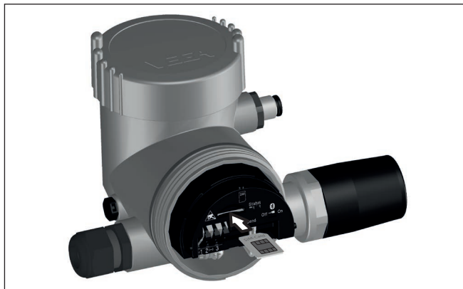
Abb. 9: Mini-SIM-Karte einsetzen
