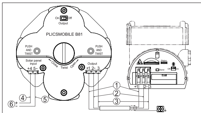
Abb. 4: Anschluss der Batterie und des Solarpanels
