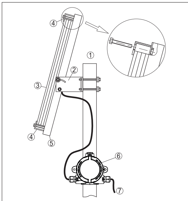
Abb. 5: Rohrmontage PLICSMOBILE mit Solarmodul
