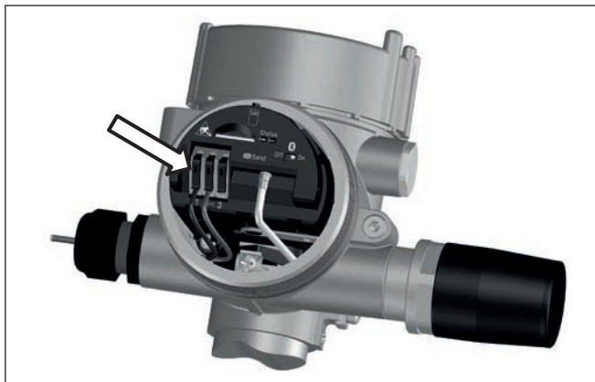
插图. 2: 接线步骤 4 和 5
