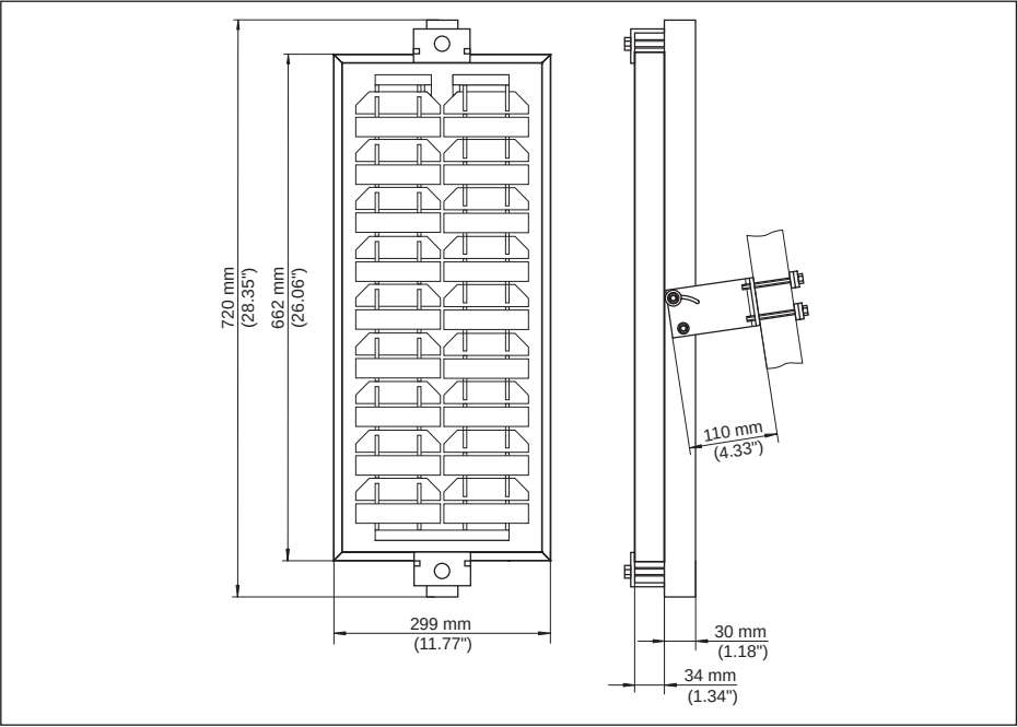
插图. 14: PLICSMOBILE S81 的尺寸
