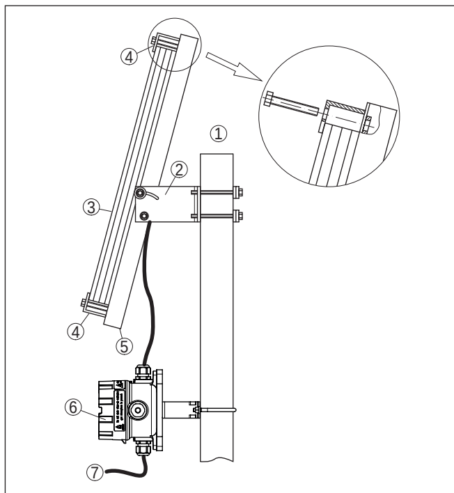
插图. 5: 将 PLICSMOBILE 通过管件式安装与太阳能电池组件相连
