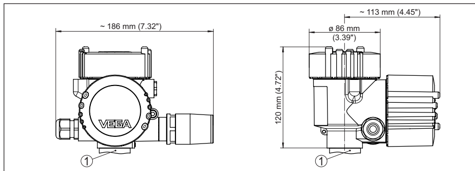
Fig. 12: Dimensions PLICSMOBILE 81 avec boîtier en aluminium/acier inoxydable
