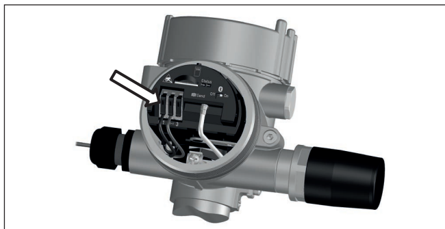
Fig. 2: Étapes de raccordement 4 et 5
