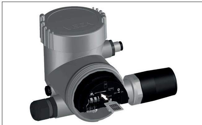
Fig. 9: Insérez la carte mini-SIM
