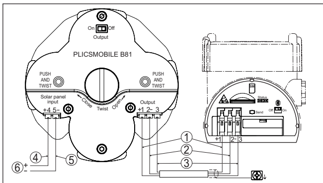
Fig. 4: Raccordement de la batterie et du panneau solaire
