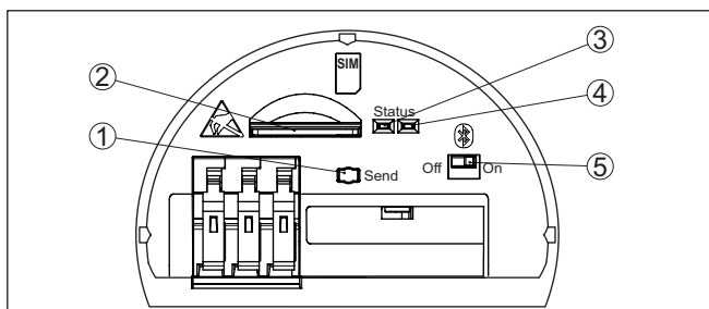
Fig. 6: Éléments de réglage et d'affichage
