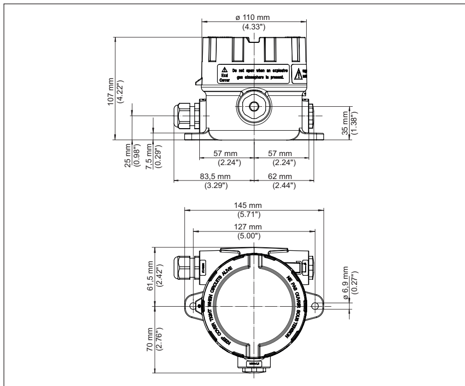
Fig. 13: Dimensions PLICSMOBILE B81 avec boîtier aluminium
