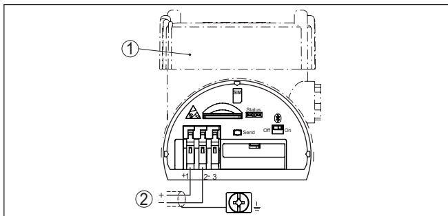
Fig. 3: Raccordement de l'alimentation tension du PLICSMOBILE 81
