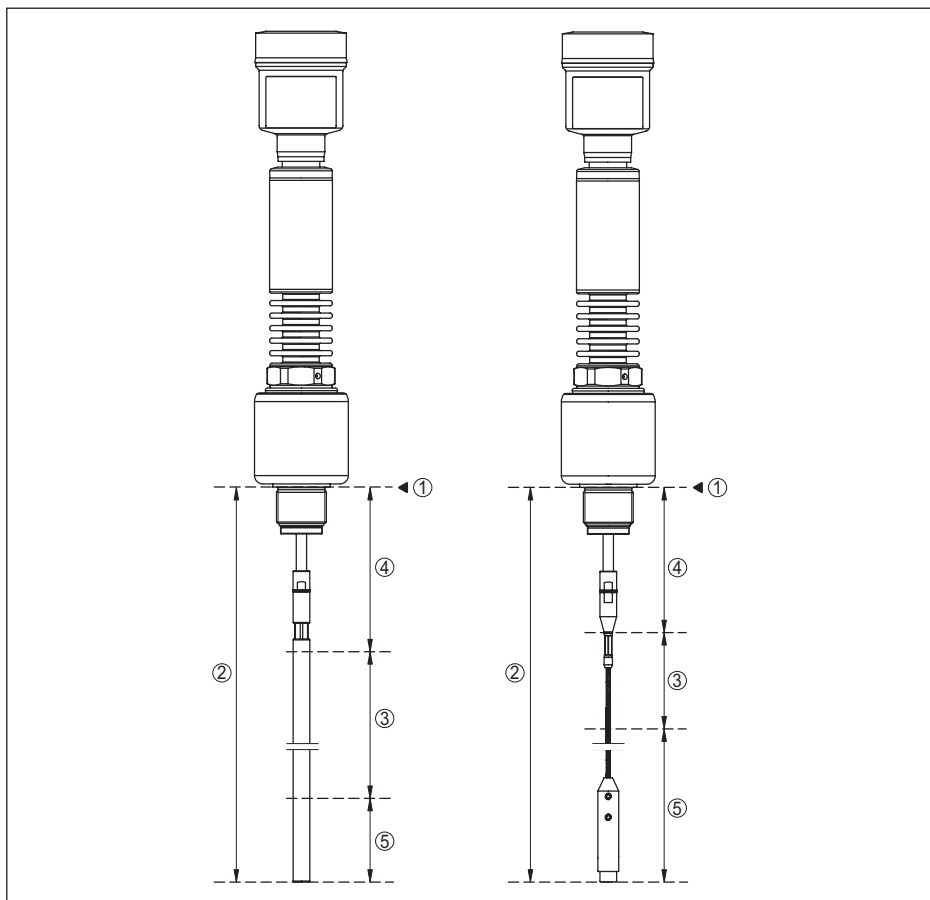
Fig. 29: Meetbereiken - VEGAFLEX 86
