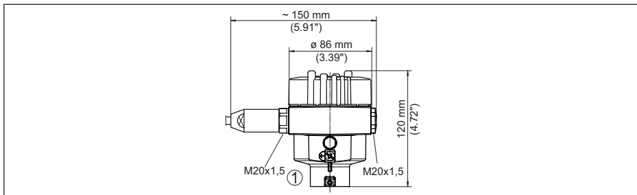
Fig. 41: Huisuitvoeringen in beschermingsklasse IP66/IP68 (1 bar), (met ingebouwde display- en bedieningsmodule wordt het huis 9 mm/0.35 in hoger)
