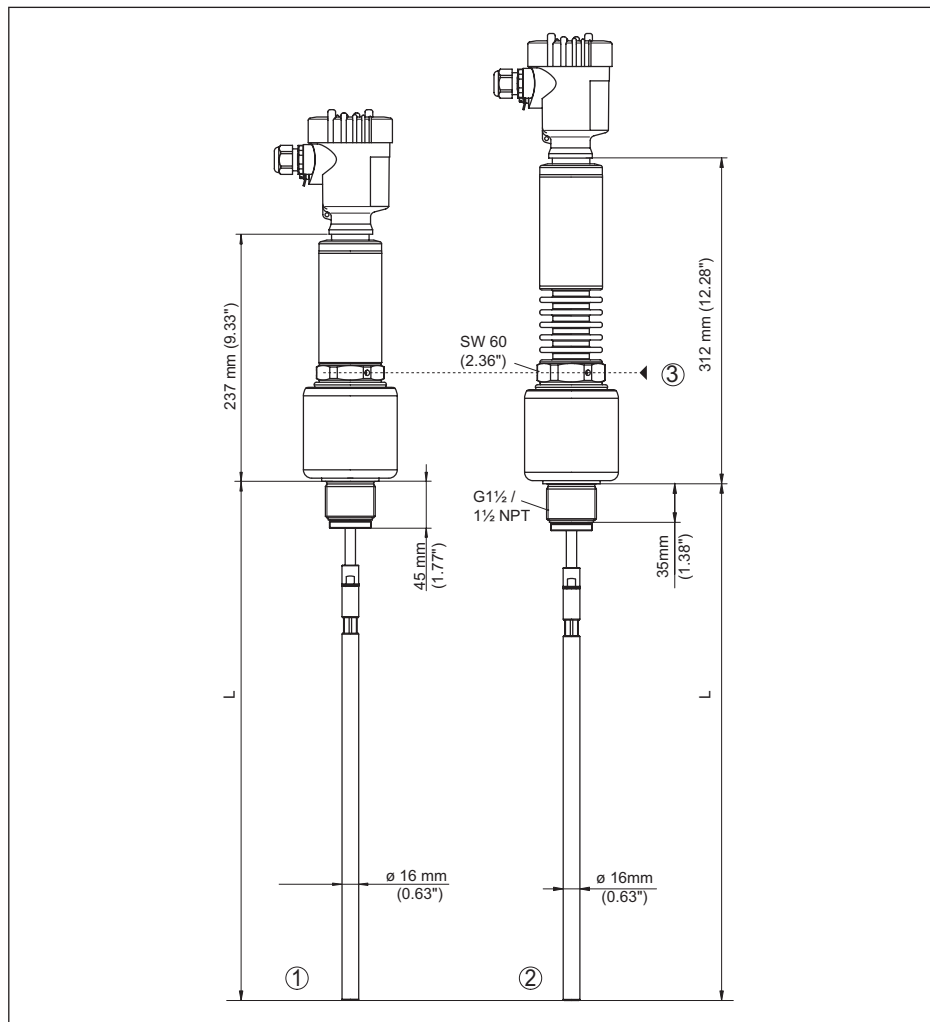
Fig. 46: VEGAFLEX 86, schroefdraaduitvoering
