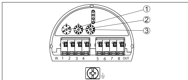
Fig. 17: Adreskeuzeschakelaar
