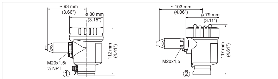
Fig. 43: Huisuitvoeringen in beschermingsklasse IP66/IP68 (1 bar), (met ingebouwde display- en bedieningsmodule wordt het huis 9 mm/0.35 in hoger)
