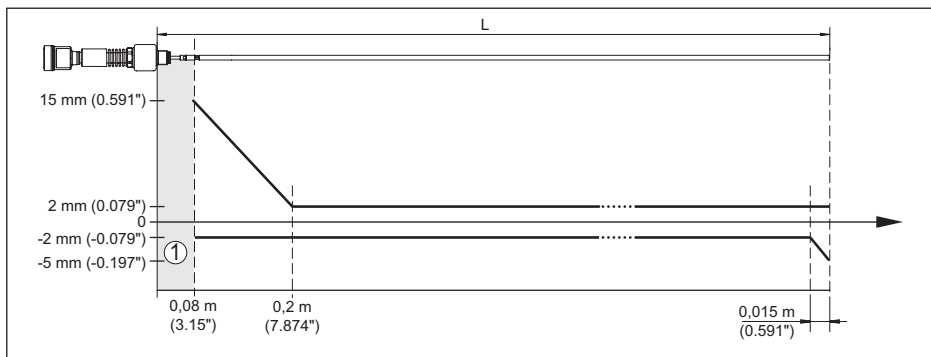
Fig. 30: Meetnauwkeurigheid VEGAFLEX 86 in staafuitvoering in medium water
