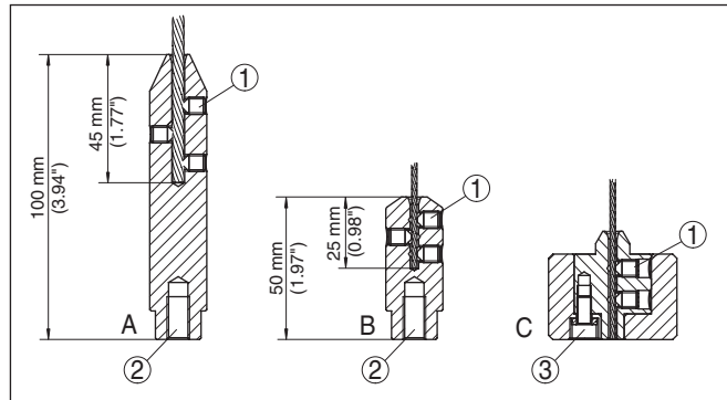
Fig. 28: Kabelmeetsonde inkorten
