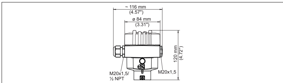
Fig. 40: Huisuitvoeringen in beschermingsklasse IP66/IP68 (0,2 bar), (met ingebouwde display- en bedieningsmodule wordt het huis 9 mm/0.35 in hoger)
