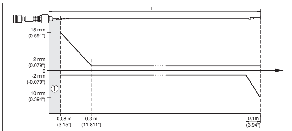
Fig. 32: Meetnauwkeurigheid VEGAFLEX 86 in kabeluitvoering in medium water
