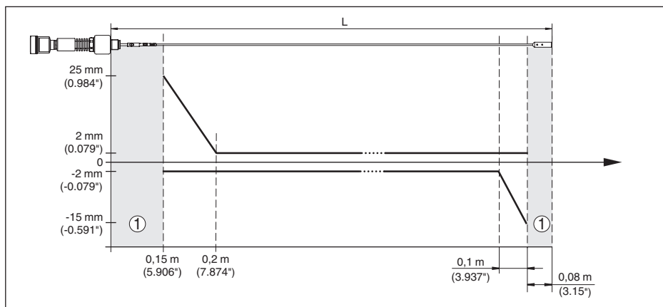
Fig. 33: Meetafwijking VEGAFLEX 86 in kabeluitvoering (2 mm/0.079 in), in medium olie
