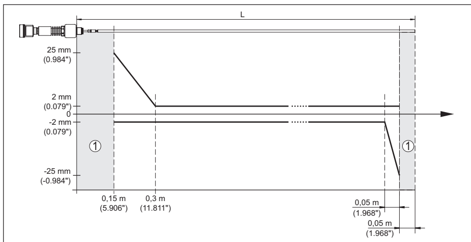
Fig. 31: Meetnauwkeurigheid VEGAFLEX 86 in staafuitvoering in medium olie
