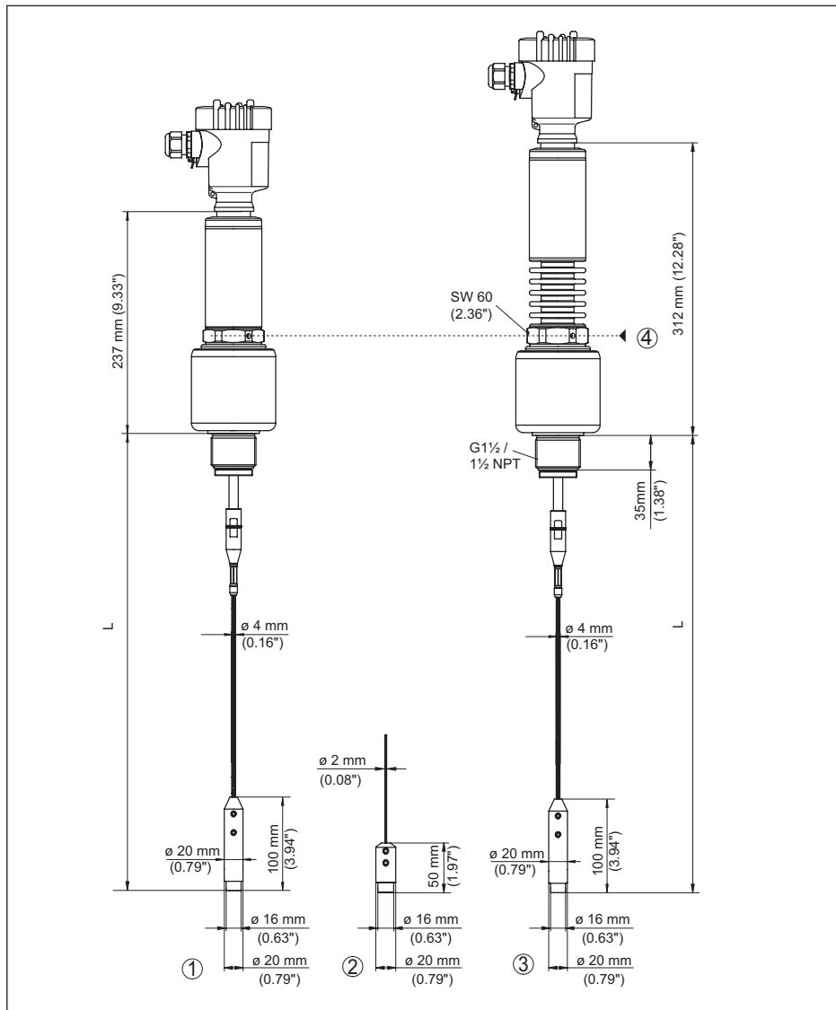
Fig. 44: VEGAFLEX 86, schroefdraaduitvoering met spangewicht (alle spangewichten met schroefdraad M8 voor oogbout)
