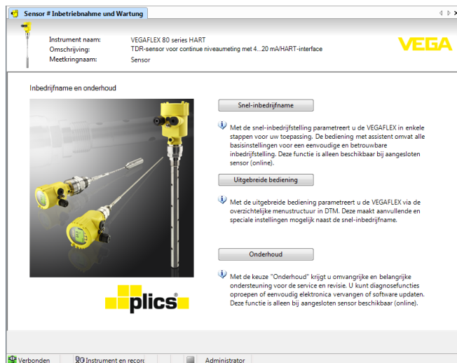
Fig. 24: Snel-inbedrijfname kiezen
