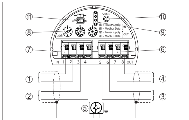
Abb. 7: Elektronikraum - Anschluss Daisy-Chain
