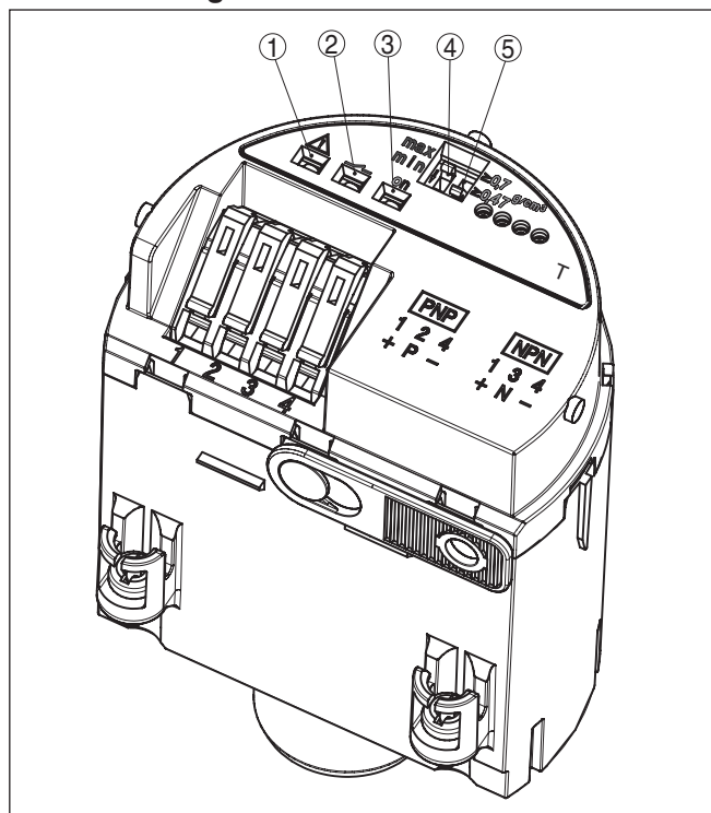
Fig. 13: Elektronica - transistoruitgang
