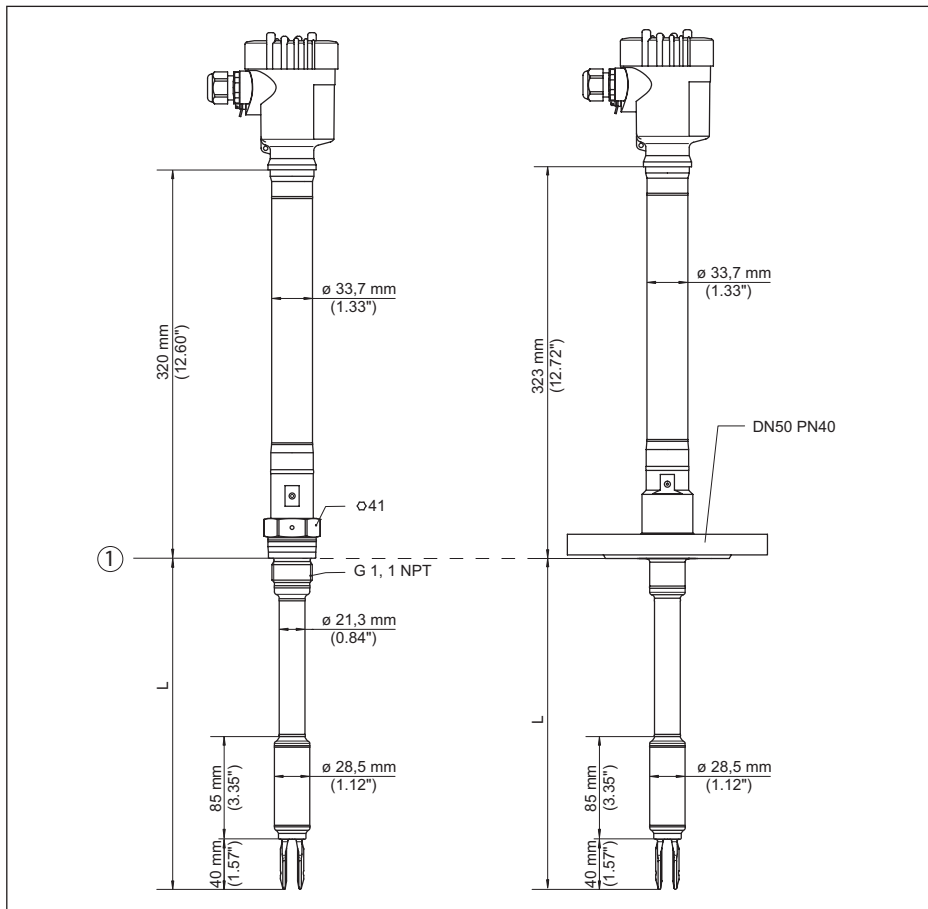
Fig. 22: VEGASWING 66, buisuitvoering
