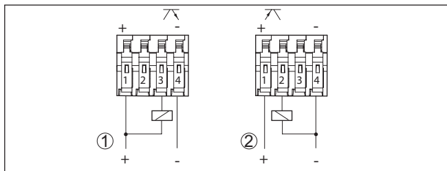
Fig. 12: Aansluitschema
