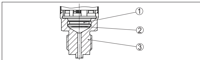
Fig. 4: Montage en retrait de la cellule de mesure (exemple : filetage G \frac{1}{2} (EN 837), raccorde de manomètre)
