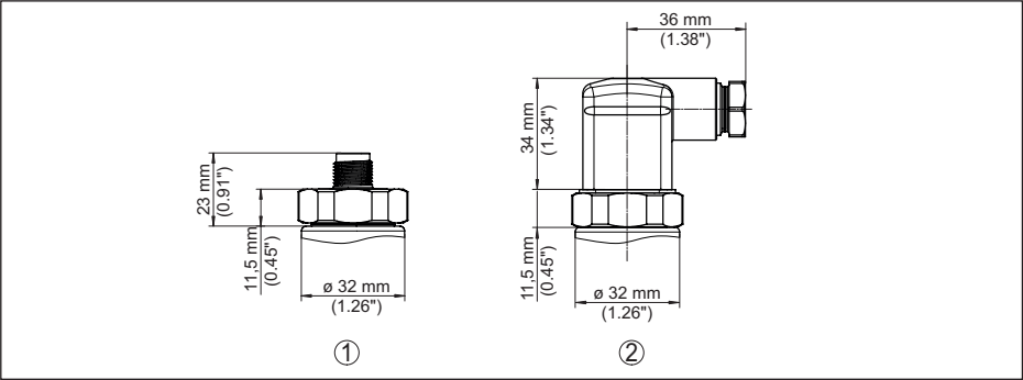
Fig. 17: Boîtier VEGABAR 19
