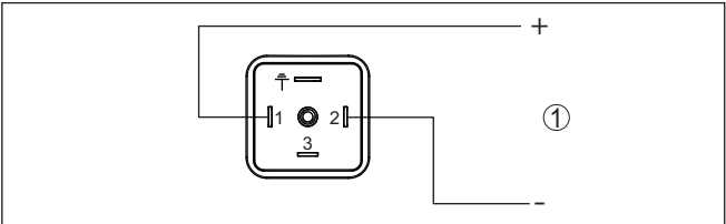
Fig. 15: Schéma de raccordement - deux fils 4 ... 20 mA - connecteur selon ISO 4400 1 Alimentation tension et sortie signal
