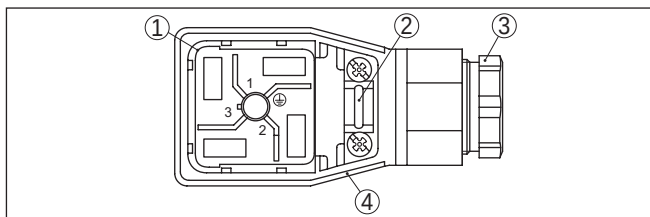
Fig. 12: Desserrez l'insert du connecteur
