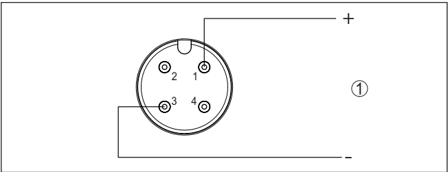
Fig. 14: Schéma de raccordement - deux fils 4 ... 20 mA - connecteur M12 x 1 1 Alimentation tension et sortie signal
