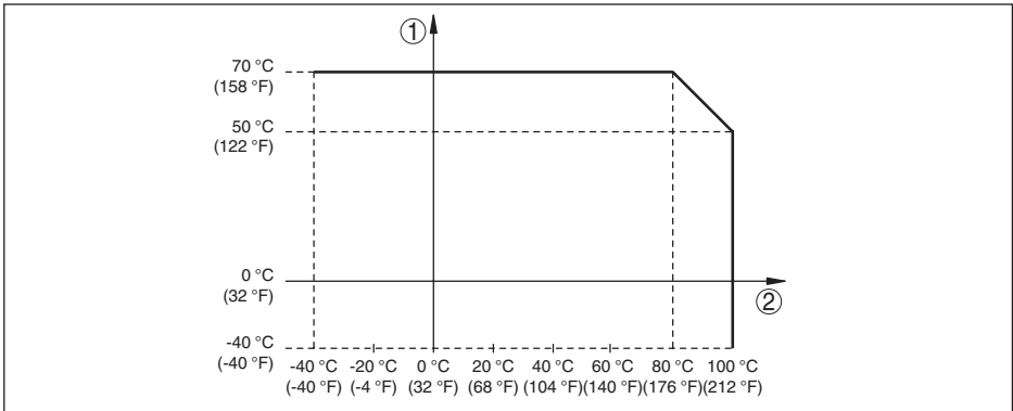
Fig. 8: Afhankelijkheid omgevingstemperatuur van processtemperatuur
