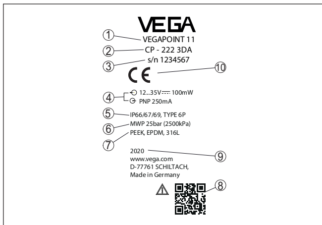
Fig. 2: Opbouw van de typeplaat (voorbeeld)
