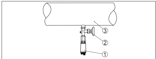
Figura 10: Configurazione di misura per la misura della pressione di processo di liquidi in tubazioni
