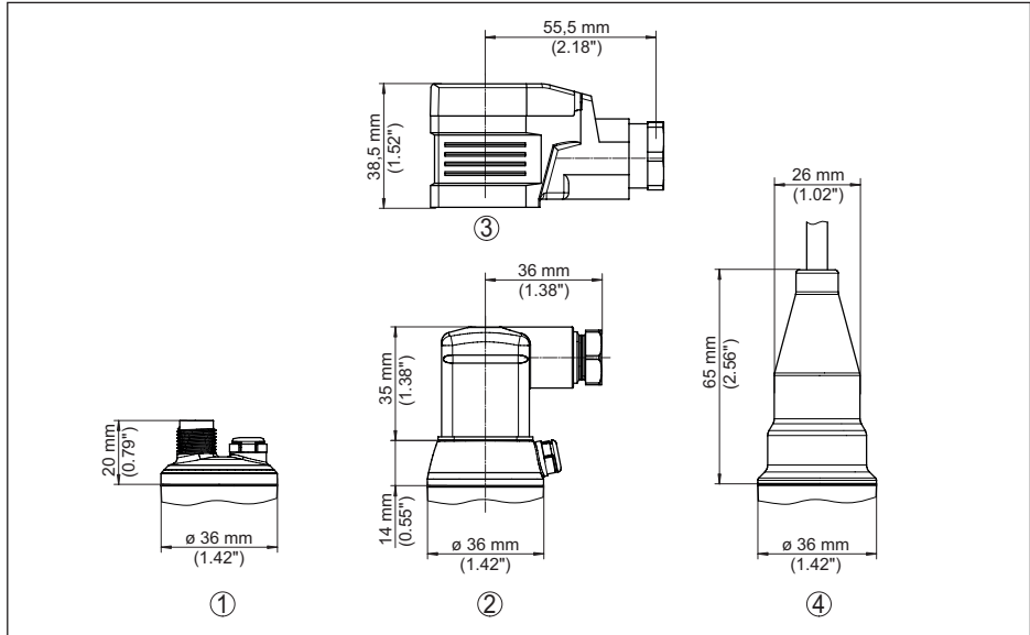
Figura 29: Tecnica di collegamento VEGABAR 29
