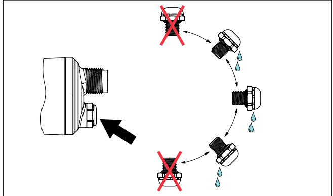
Figura 6: Orientamento del filtro
