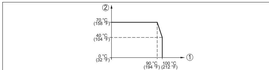
Figura 28: Derating termico VEGABAR 29, con comunicazione Bluetooth attivata
