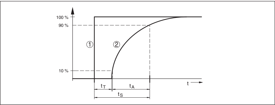
Fig. 25: Gedrag van de stroomuitgang bij sprongsgewijze verandering van de proceseenheid. t_T : dode band; t_A : toenametijd; t_s : sprongantwoordtijd
