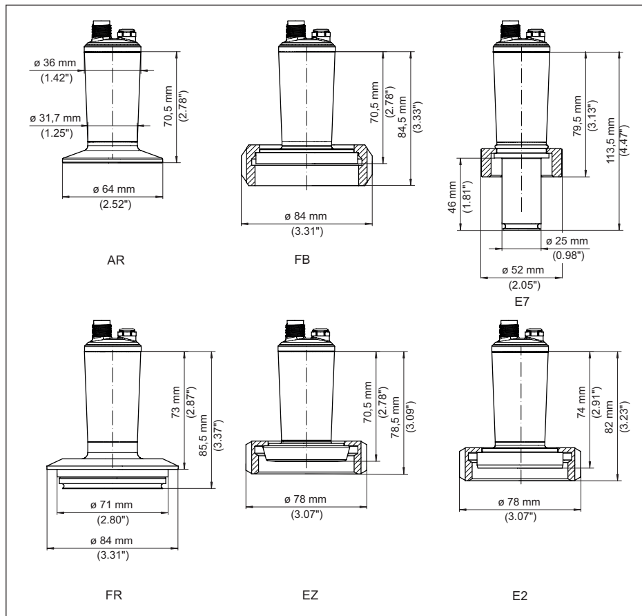
Fig. 33: VEGABAR 29, aseptische aansluiting
