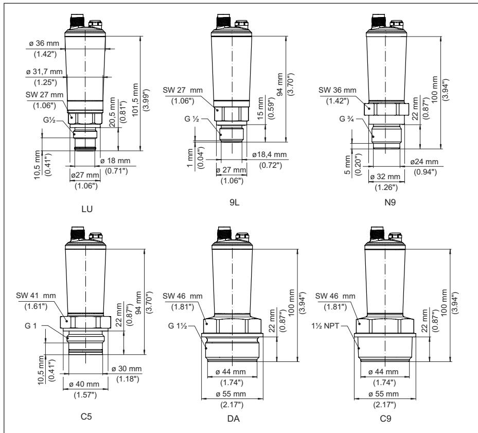
Fig. 31: VEGABAR 29, schroefdraadaansluiting vlak
