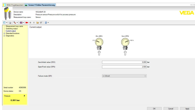
Fig. 23: Voorbeeld van een DTM-aanzicht - inregeling stroomuitgang
