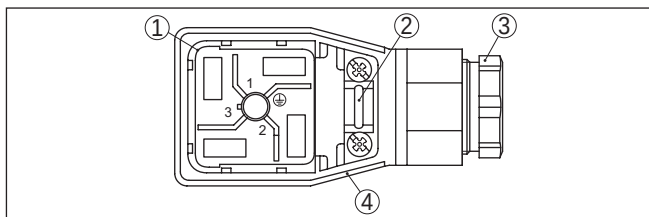
Fig. 14: Losmaken van het binnenwerk.
