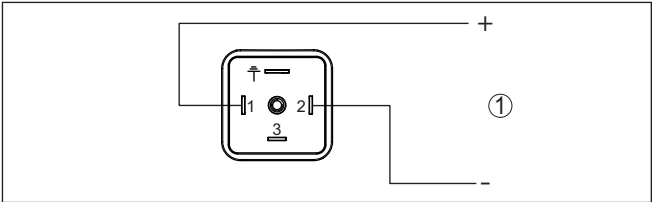
Fig. 18: Aansluitschema - tweedraads 4 ... 20 mA - stekker conform ISO 4400 1 Voedingsspanning en signaaluitgang
