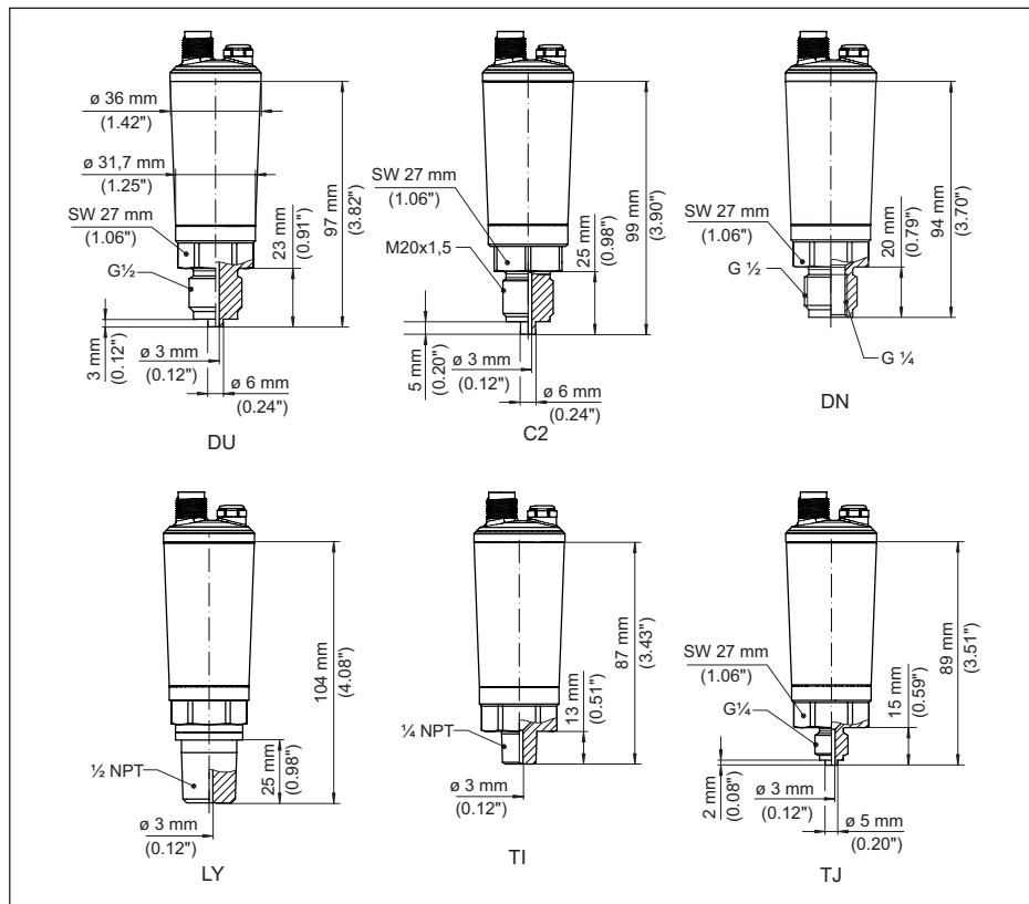
Fig. 30: VEGABAR 29, schroefdraadaansluiting niet vlak
