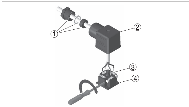
Fig. 13: Aansluiting op de schroefklemmen
