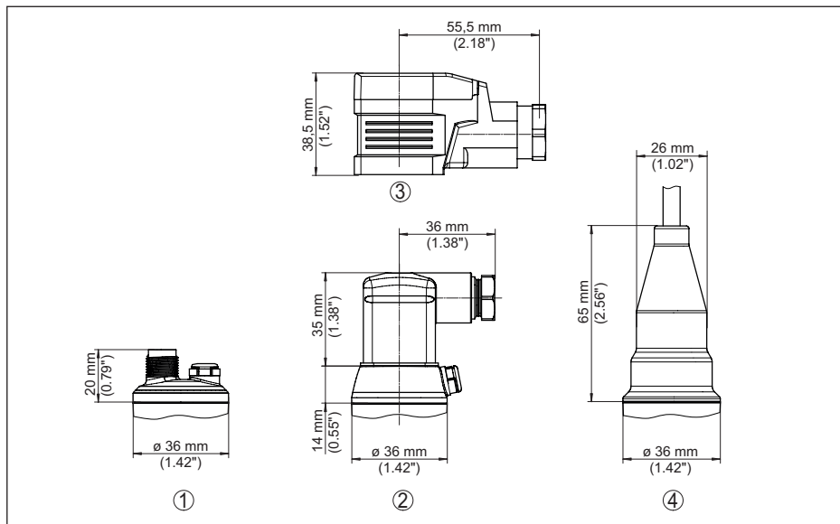
Fig. 29: Aansluittechniek VEGABAR 29
