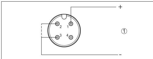
Fig. 17: Aansluitschema - tweedraads 4 ... 20 mA - M12 x 1-stekker
