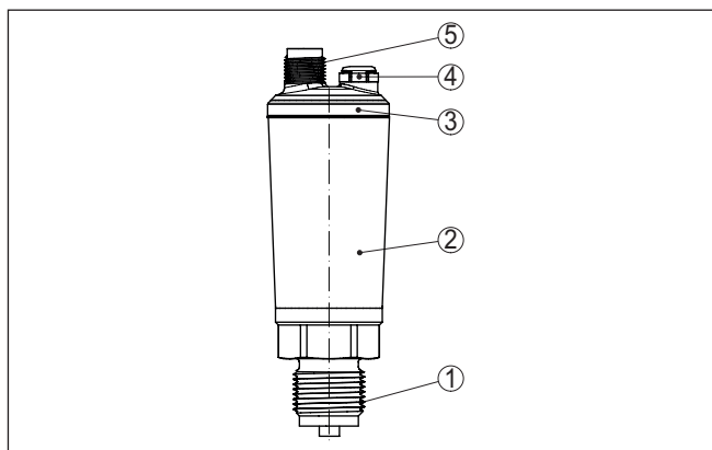
Fig. 1: Componenten van de VEGABAR 29
