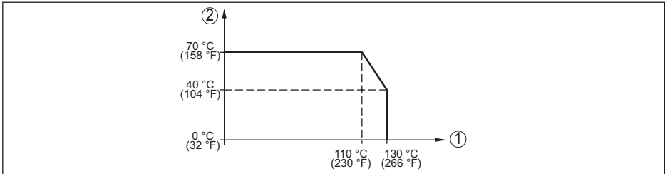
Fig. 27: Temperatuurderating VEGABAR 29
