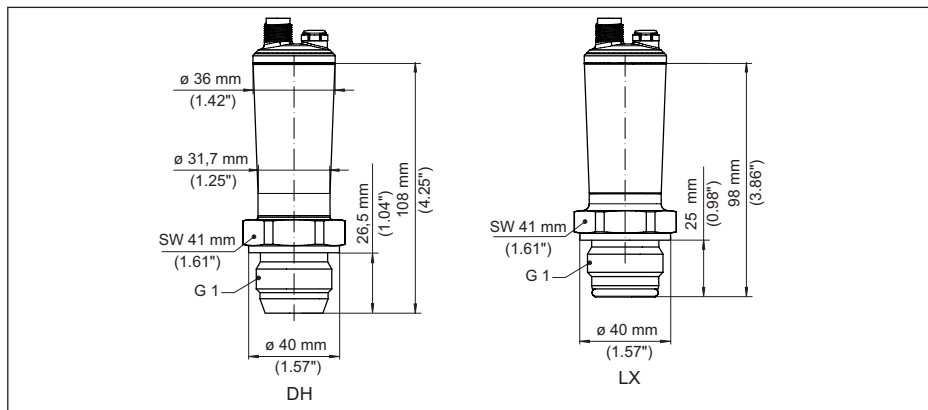
Fig. 32: VEGABAR 29, conus-/tubusaansluiting
