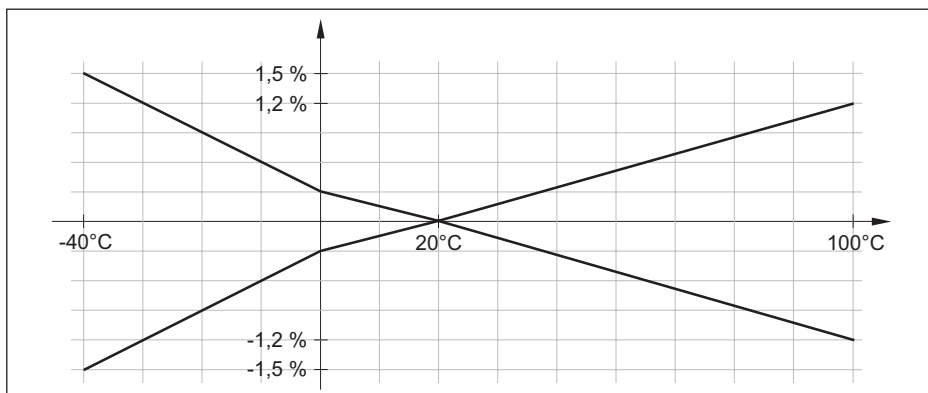
Fig. 26: Temperatuurfout bij TD 1 : 1
