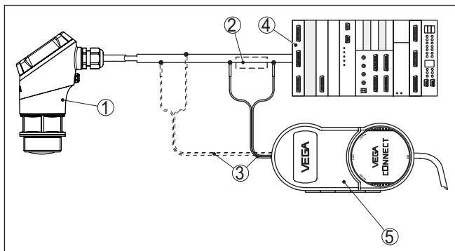
Fig. 29: Aansluiting van de PC op de signaalkabel
