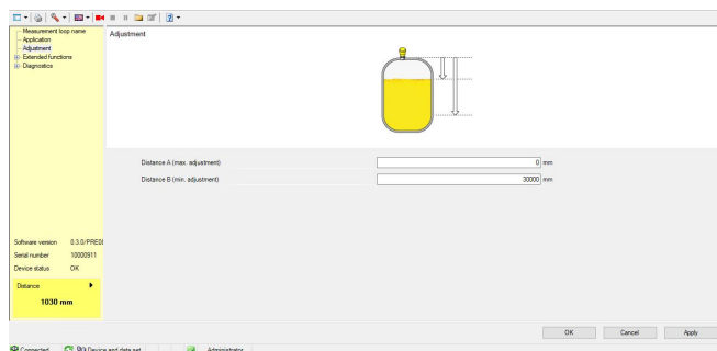
Fig. 31: Voorbeeld van een DTM-aanzicht
