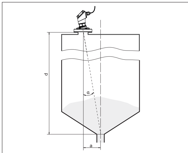
Fig. 14: Voorstel voor de inbouw na uitrichting VEGAPULS 31
