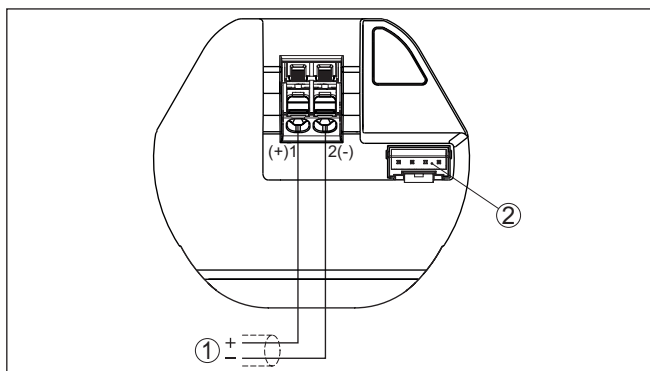
Fig. 19: Aansluitruimte VEGAPULS 31
