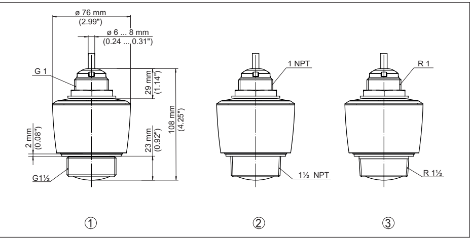
Fig. 31: Encombrement VEGAPULS C 21
