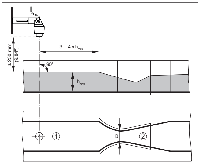
Fig. 18: Mesure du débit avec canal Venturi Khafagi : h_{\text{max}} = remplissage max. du canal ; B = resserrement max. du canal
