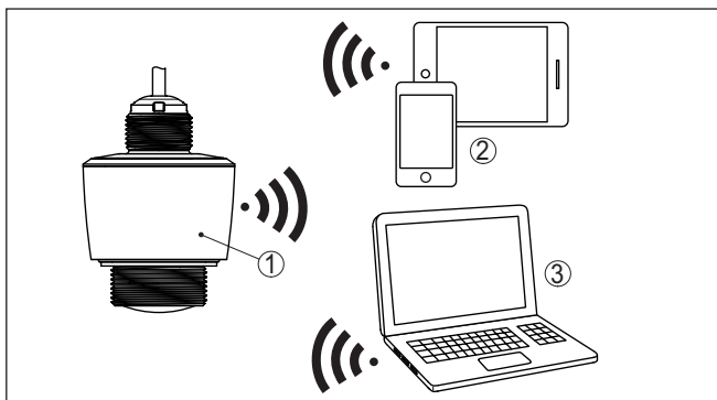
Fig. 2: Connexion sans fil aux outils de réglage standard avec Bluetooth intégré LE
