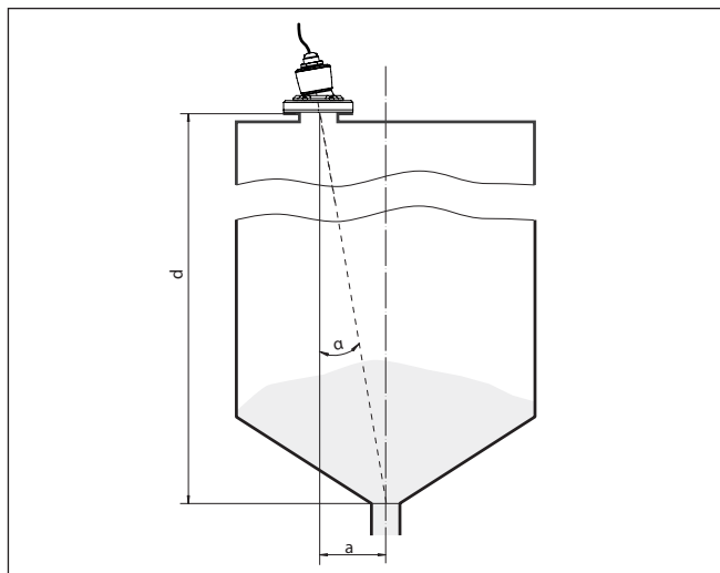
Fig. 15: Proposition pour un montage après orientation VEGAPULS C 21
