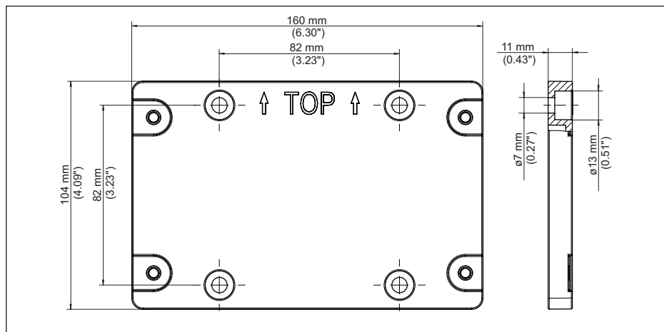
Abb. 23: Maße Montageplatte
