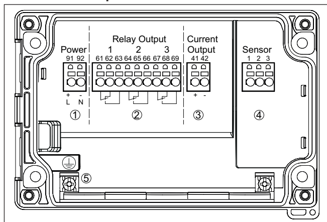
Abb. 6: Anschlussplan VEGAMET 841
