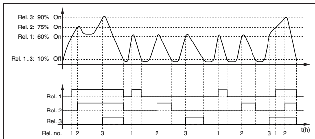
Abb. 18: Beispiel für Pumpensteuerung 4
