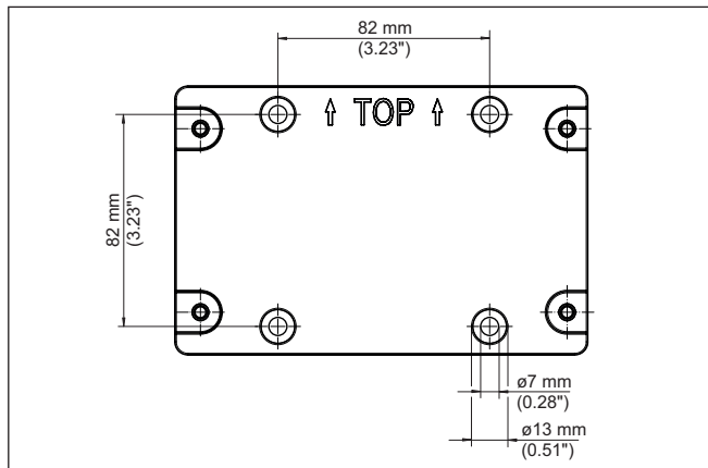
Abb. 3: Montageplatte für Wandmontage VEGAMET 841
