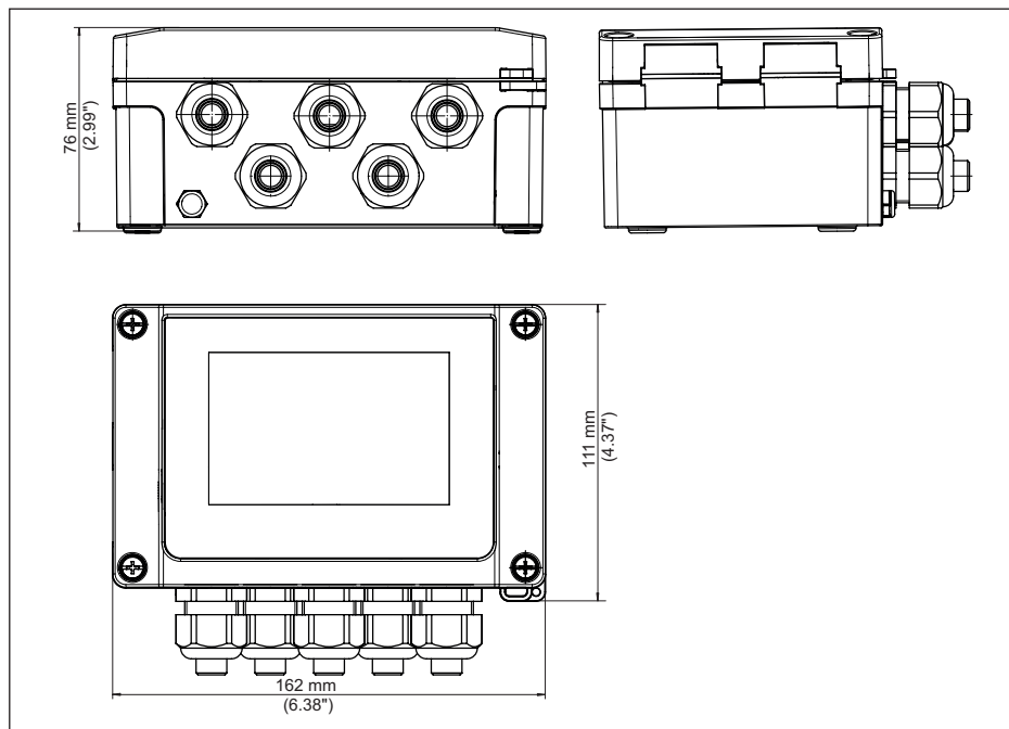
Abb. 22: Maße VEGAMET 841
