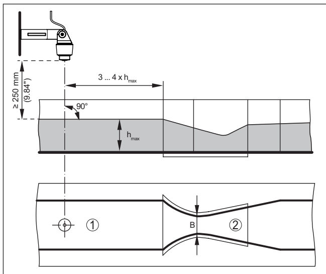
Abb. 21: Durchflussmessung mit Khafagi-Venturirinne: h_{max} = max. Befüllung der Rinne; B = größte Einschnürung der Rinne
