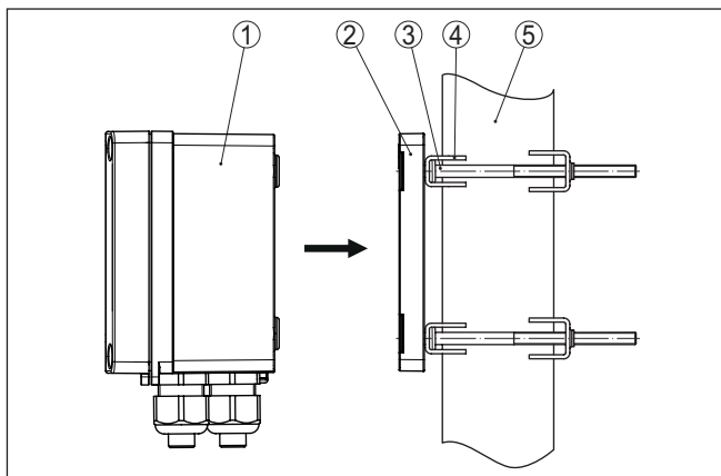
Abb. 4: Rohrmontage
