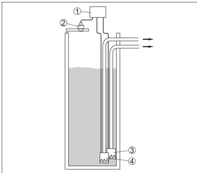
Abb. 14: Beispiel Pumpstation: Pumpensteuerung im Einlaufschacht
