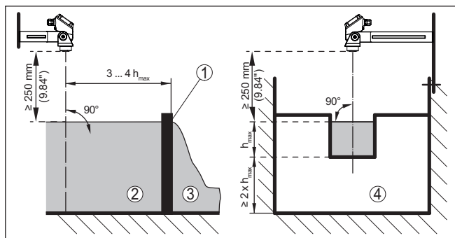
Figura 20: Misura di portata con stramazzo rettangolare: h_{\text{max}} = max. riempimento dello stramazzo rettangolare
