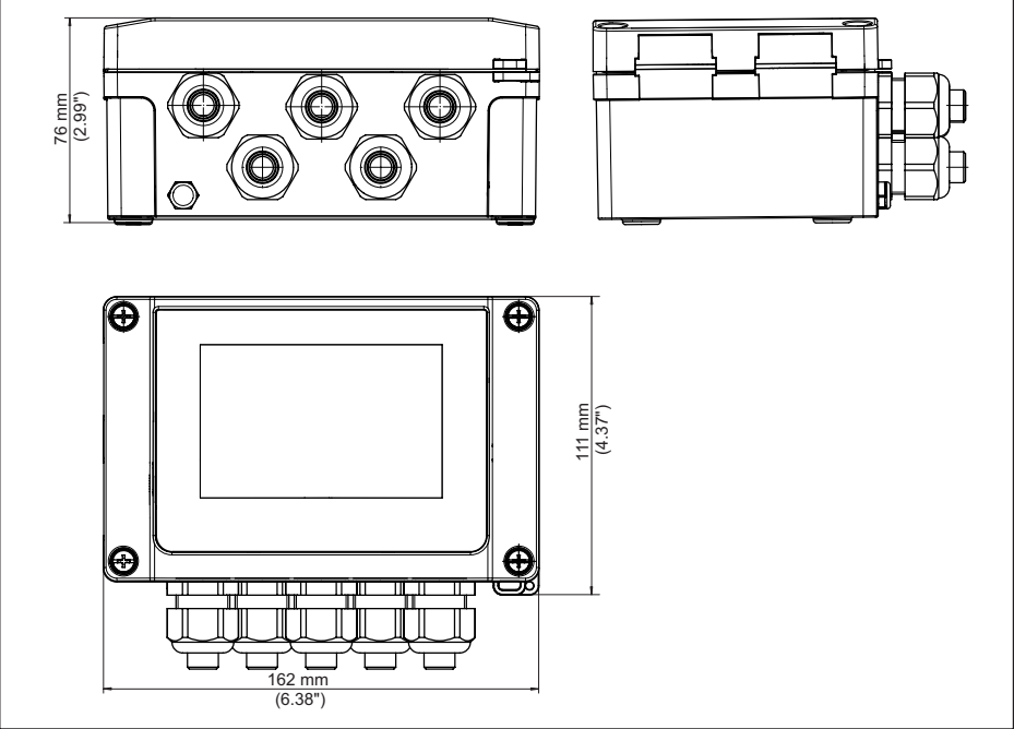
Figura 22: Dimensioni VEGAMET 841
