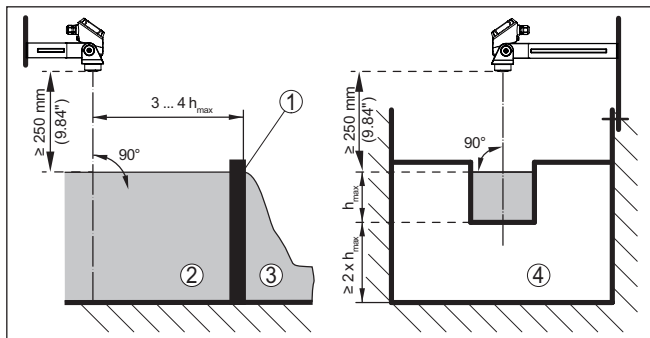
Figura 20: Misura di portata con stramazzo rettangolare: h_{\max.} = \max. riempimento dello stramazzo rettangolare
