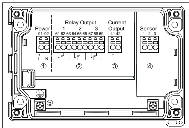
Fig. 6: Aansluitschema VEGAMET 841
