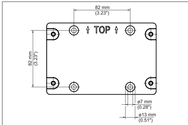
Fig. 3: Montageplaat voor wandmontage VEGAMET 841
