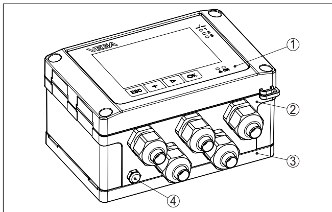
Fig. 1: VEGAMET 841
