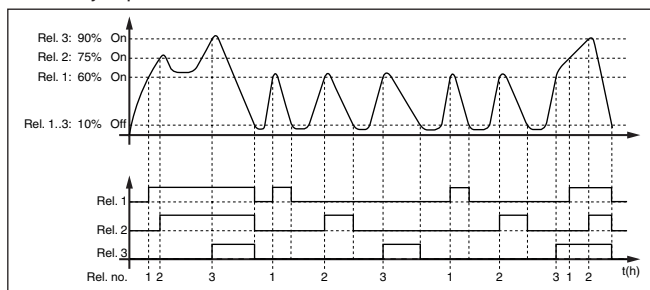
Fig. 18: Ejemplo de control de bomba 4
