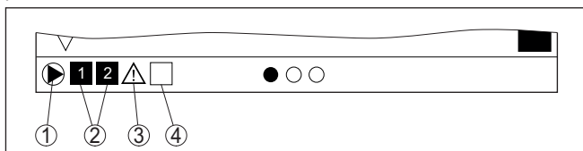
Fig. 15: Barra de estado en la pantalla cuando se activa el control de la bomba
