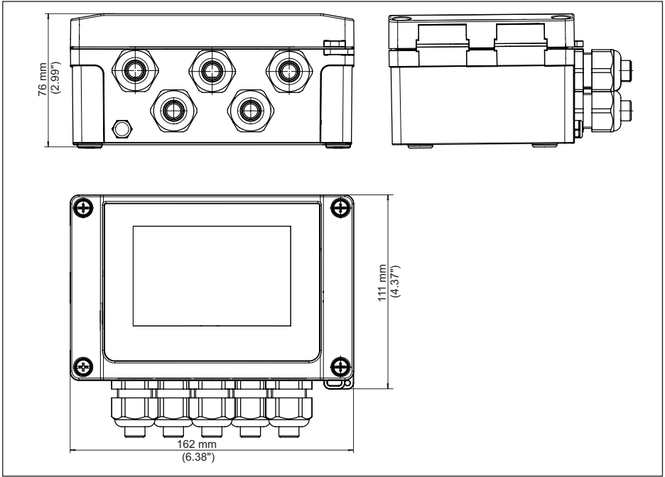
Fig. 22: Medidas VEGAMET 841
