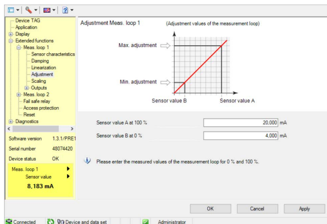
Figura 14: Esempio di schermata DTM - Taratura
