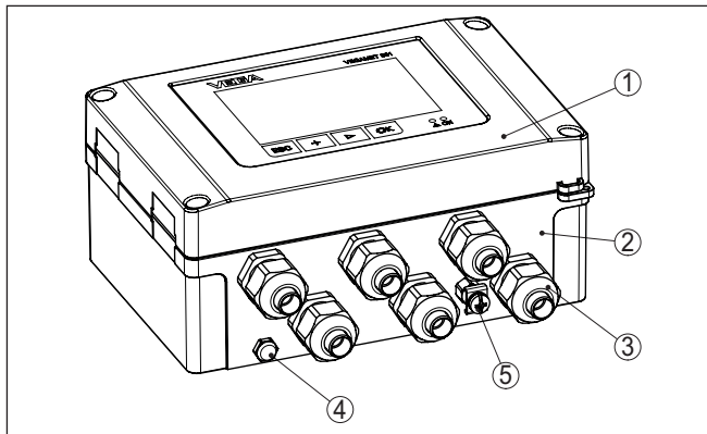
Figura 1: VEGAMET 861
