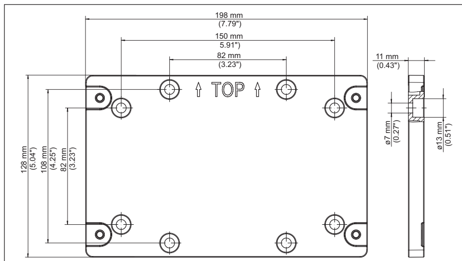
Fig. 25: Afmetingen montageplaat
