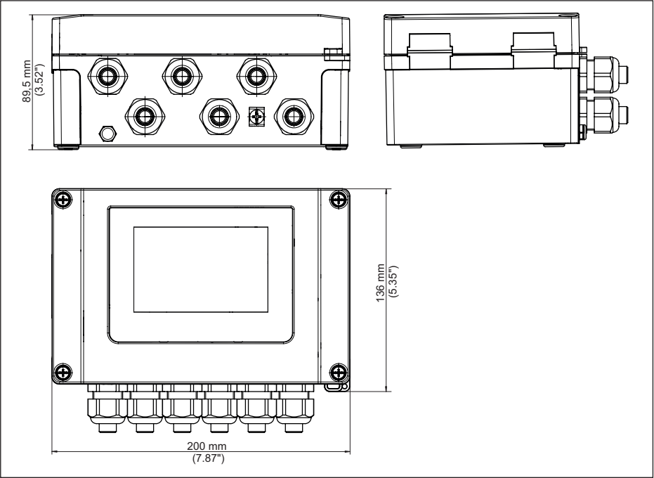
Fig. 24: Afmetingen VEGAMET 861
