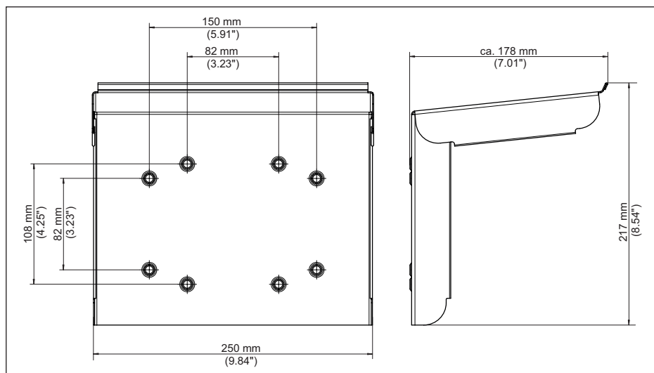
Fig. 26: Afmetingen zonnedak
