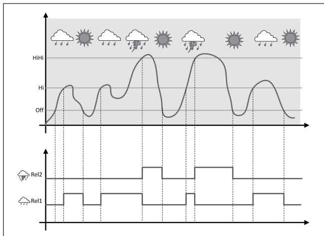
Fig. 21: Voorbeeld van een pompregeling met optie "mooiweerbij"
