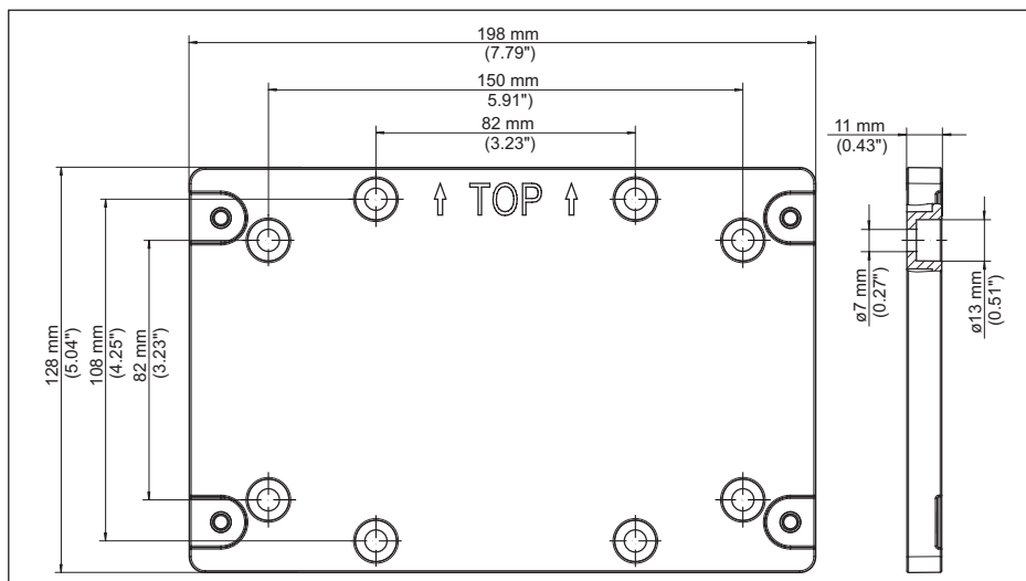
Fig. 25: Afmetingen montageplaat
