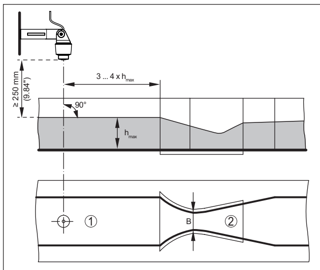
Fig. 23: Flowmeting met Khafagi-venturigoot: h_{max} = max. peil in de goot; B = maximale insnoering van de goot
