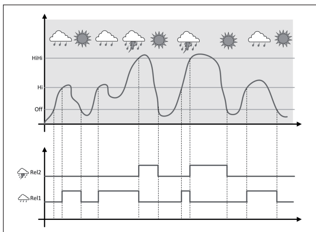
Fig. 19: Voorbeeld van een pompregeling met optie "mooiweerbetrieb"
