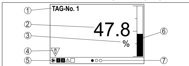
Fig. 11: Voorbeeld meetwaarde-indicatie (meetwaarde met bargraph)
