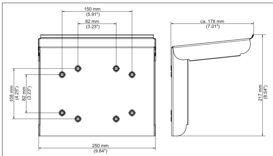
Fig. 26: Afmetingen zonnedak
