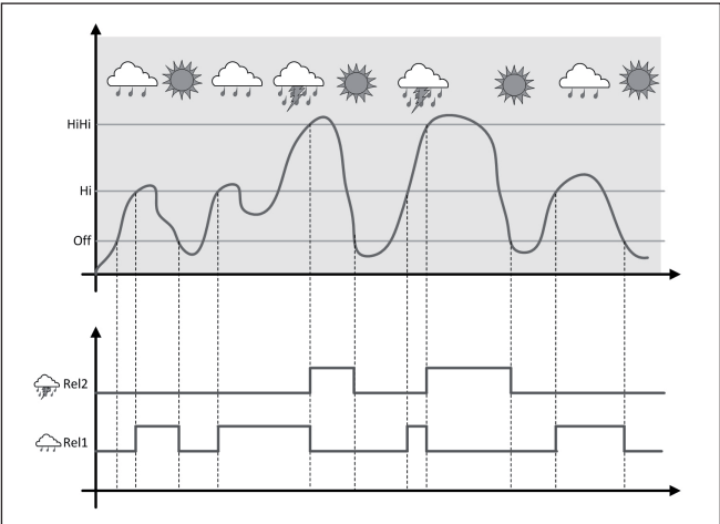
Fig. 21: Voorbeeld van een pompregeling met optie "mooiweerbedrijf"
