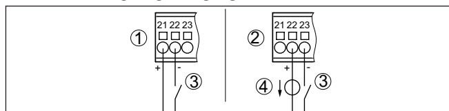
Fig. 9: Aansluitbezetting van de digitale ingangen (actief/passief)
