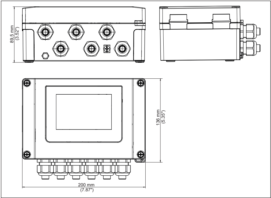
Fig. 24: Afmetingen VEGAMET 861
