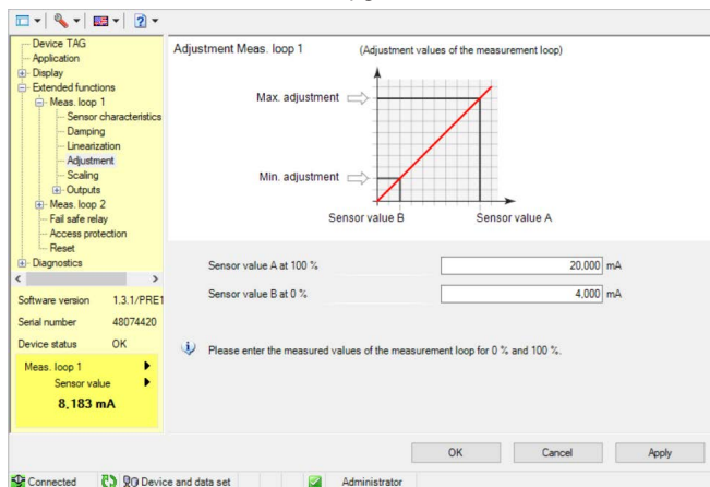
Fig. 14: Voorbeeld van een DTM-aanzicht - Inregeling
