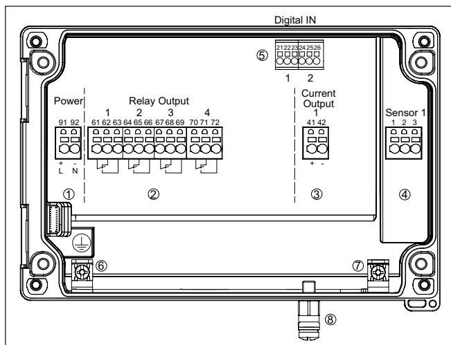
Fig. 6: Aansluitschema VEGAMET 861
