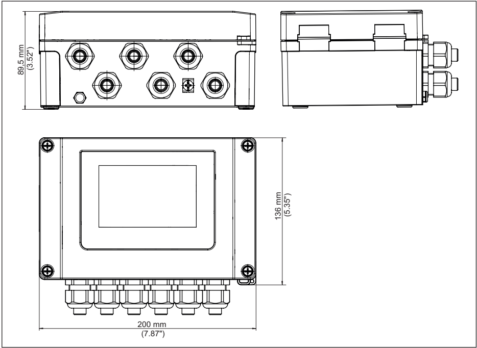
Fig. 24: Medidas VEGAMET 861
