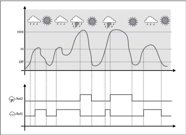
Fig. 21: Ejemplo de un control de bombas con la opción "Operación de buen tiempo"
