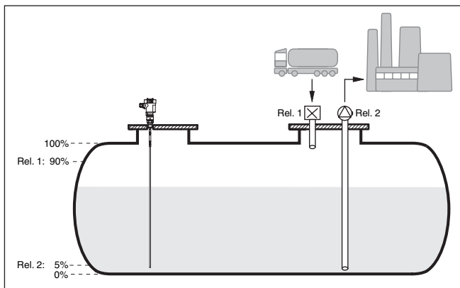
Fig. 15: Ejemplo de medida de nivel tanque en cilíndrico horizontal
