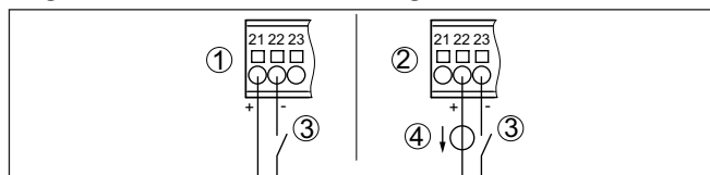
Fig. 9: Asignación de conexión de las entradas digitales (activa/pasiva)
