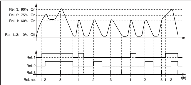
Fig. 20: Ejemplo de control de bomba 4
