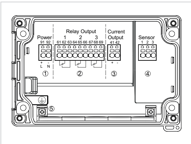
Aansluitschema VEGAMET 841
