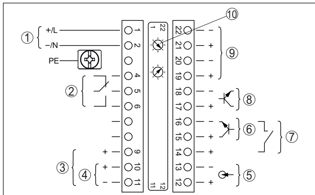
Fig. 10: Elektronica- en aansluitruimte bij niet-Ex instrumenten en instrumenten met niet-intrinsiekveilige stroomuitgang
