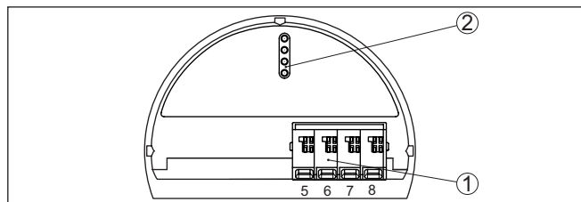
Fig. 11: Bedienings- en aansluitruimte bij niet-Ex instrumenten en instrumenten met niet-intrinsiekveilige signaaluitgang
