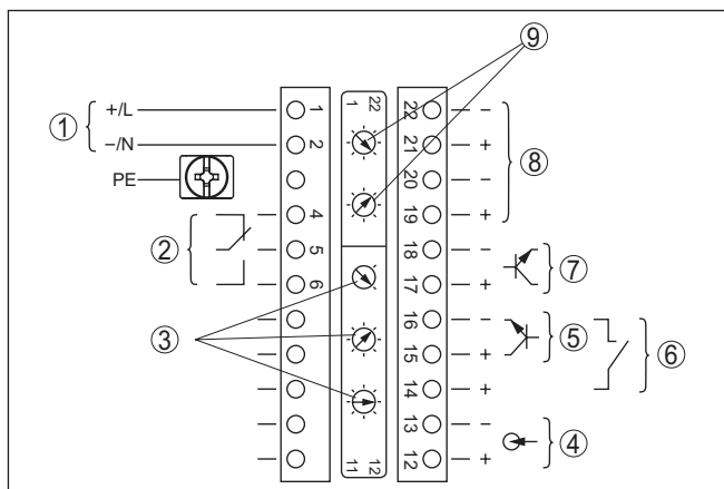
Fig. 12: Elektronica- en aansluitruimte (Ex-d) bij instrumenten met intrinsiekveilige signaaluitgang
