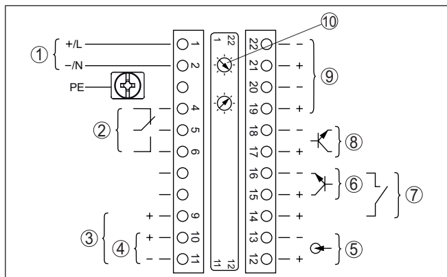
Fig. 8: Elektronica- en aansluitruimte bij niet-Ex instrumenten en instrumenten met niet-intrinsiekveilige stroomuitgang
