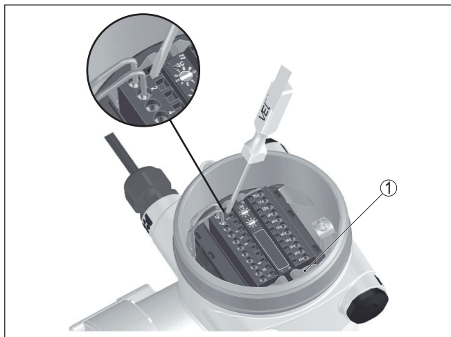
Abb. 7: Anschlussschritte 4 und 5
