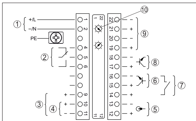
Abb. 8: Elektronik- und Anschlussraum bei Nicht-Ex-Geräten und Geräten mit nicht-eigensicherem Stromausgang
