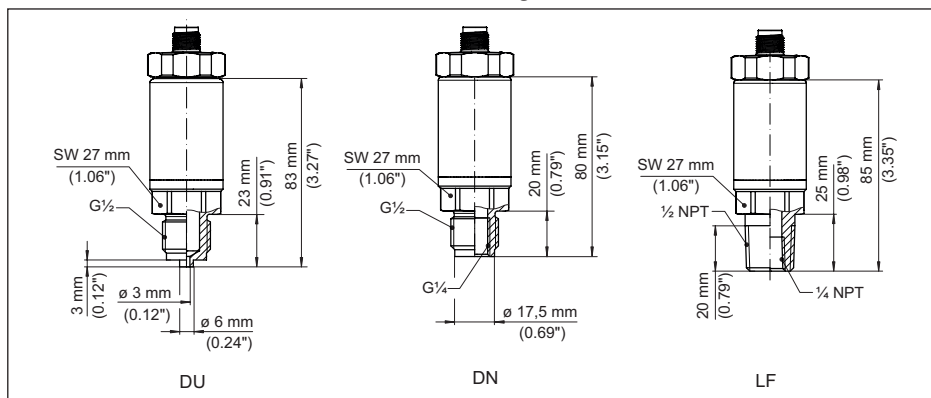
Abb. 17: VEGABAR 18, Gewindeanschluss nicht frontbündig
