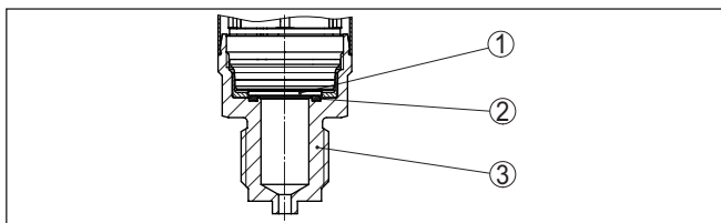
Abb. 5: Zurückgesetzter Einbau der Messzelle (Beispiel: Gewinde G\frac{1}{2} , EN 837 Manometeranschluss)
