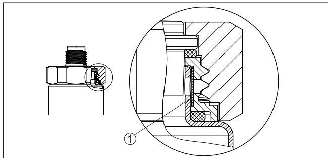
Abb. 6: Position des Filterelementes
