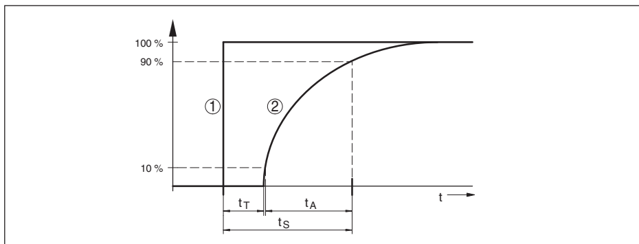
Abb. 15: Verhalten des Stromausganges bei sprunghafter Änderung der Prozessgröße. t_T : Totzeit; t_A : Anstiegszeit; t_S : Sprungantwortzeit
