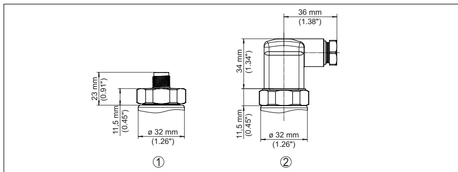
Abb. 16: Gehäuse VEGABAR 18
