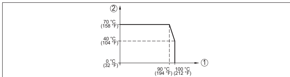
Fig. 32: Derating de température VEGABAR 38, avec la communication Bluetooth activée
