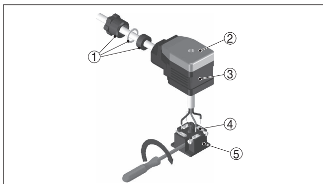
Fig. 17: Raccordement aux bornes à vis
