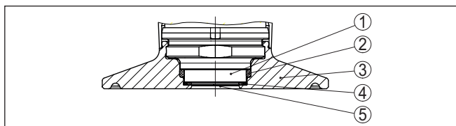
Fig. 6: Montage hygiénique de la cellule de mesure (exemple : Clamp 2")
