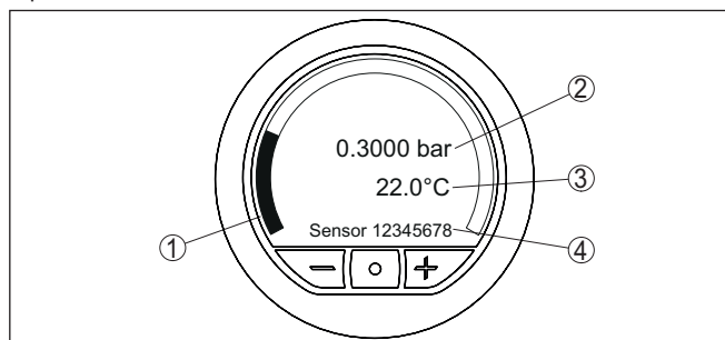
Fig. 22: Affichage de la valeur mesurée avec des affichages supplémentaires
