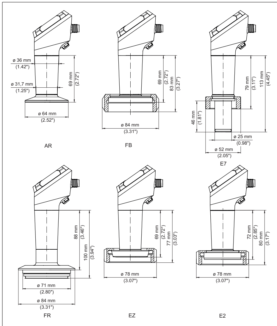
Fig. 37: VEGABAR 38, raccord aseptique
