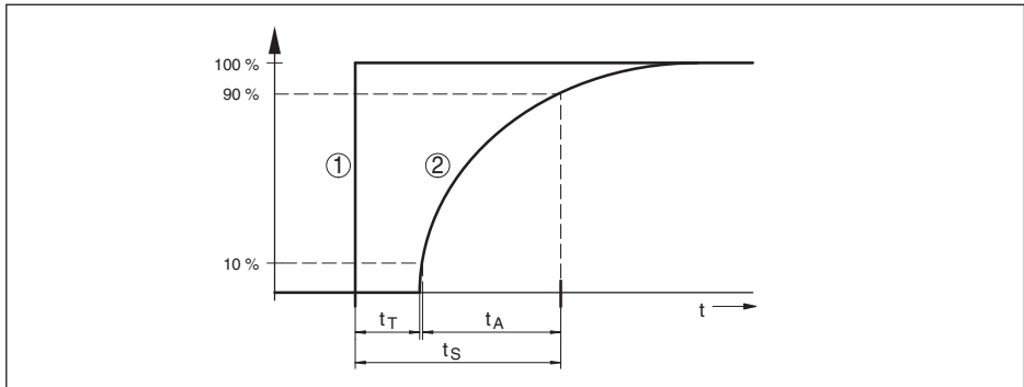
Fig. 29: Comportement du courant de sortie en cas de variation brusque de la grandeur process. t_T : temps mort ; t_A : temps de montée ; t_s : temps de réponse impulsionnelle
