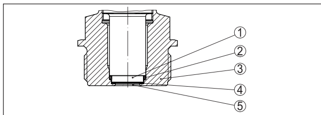
Fig. 5: Montage arasant de la cellule de mesure (exemple : filetage G1½)
