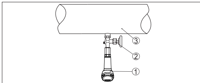
Fig. 12: Mise en œuvre pour la mesure de pression process de liquides dans des conduites
