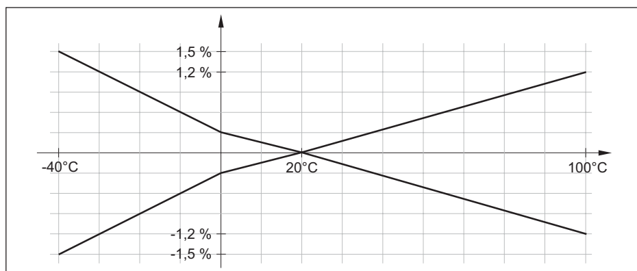
Fig. 30: Erreur de température avec TD 1 : 1
