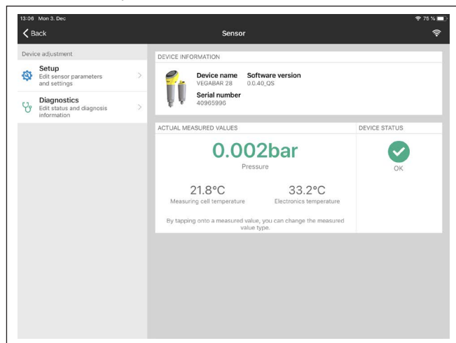
Fig. 25: Exemple de vue de l'appli - Mise en service valeurs mesurées
