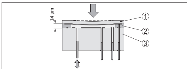
Fig. 3: Structure de la cellule de mesure Mini-CERTEC®
