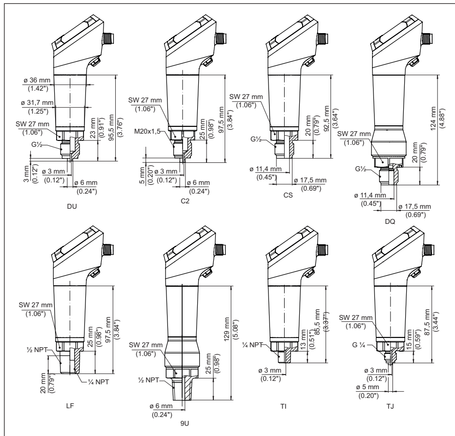
Fig. 34: VEGABAR 38, raccord fileté non arasant
