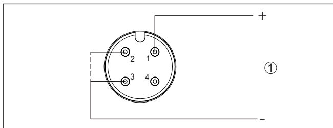
Fig. 20: Schéma de raccordement - deux fils 4 ... 20 mA - connecteur M12 x 1 1 Alimentation tension et sortie signal
