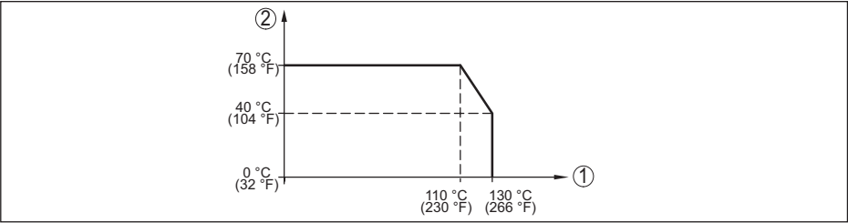
Fig. 31: Derating de température VEGABAR 38
