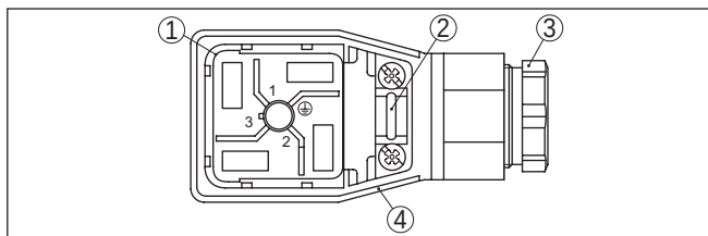
Fig. 16: Desserrez l'insert du connecteur
