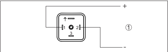
Fig. 19: Schéma de raccordement - deux fils 4 ... 20 mA - connecteur selon ISO 4400
