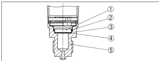
Fig. 4: Montage en retrait de la cellule de mesure (exemple : filetage G½ (EN 837), raccorde de manomètre)
