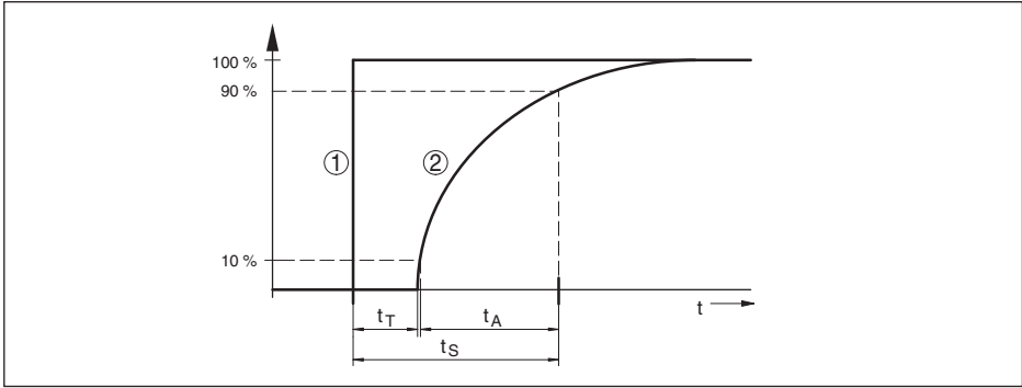
Fig. 32: Comportement du courant de sortie en cas de variation brusque de la grandeur process. t_T : temps mort ; t_A : temps de montée ; t_S : temps de réponse impulsionnelle
