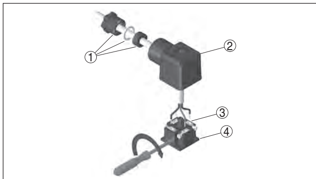
Fig. 14: Raccordement aux bornes à vis
