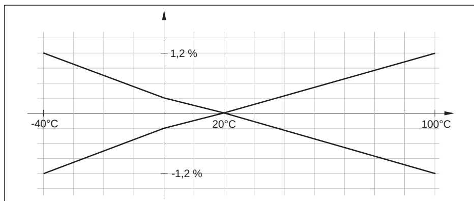
Fig. 29: Erreur de température avec TD 1 : 1
