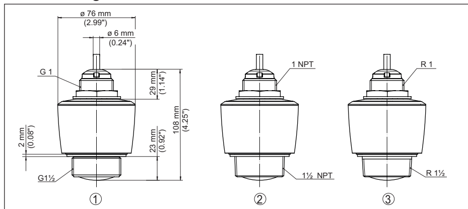
Fig. 27: Afmetingen VEGAPULS C 11
