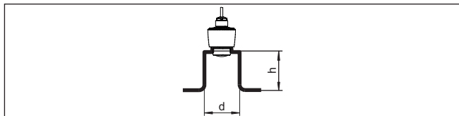
Fig. 10: Sokmontage bij afwijkende afmetingen
