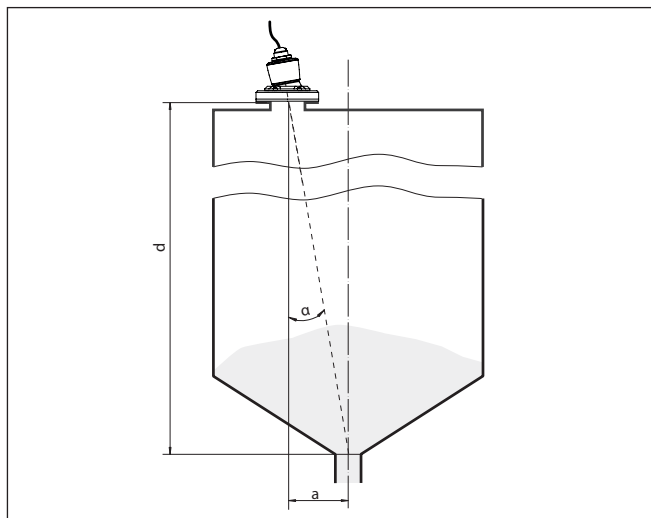
Fig. 14: Voorstel voor de inbouw na uitrichting VEGAPULS C 11
