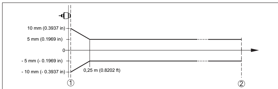
Fig. 26: Meetnauwkeurigheid onder referentiecondities 7)
