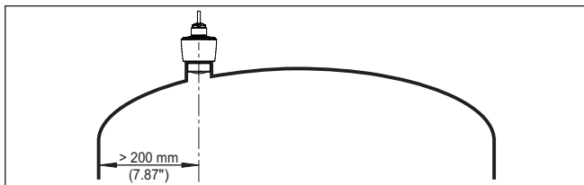
Fig. 5: Montage van de radarsensor op ronde tankdaken
