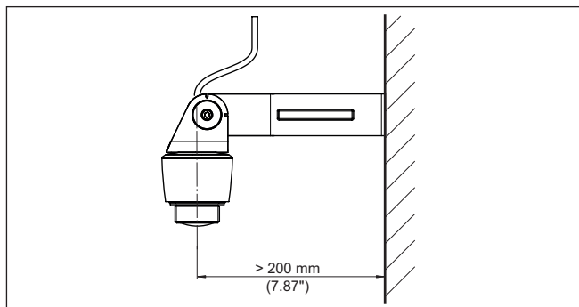
Fig. 3: Montage via een montagehoekstuk
